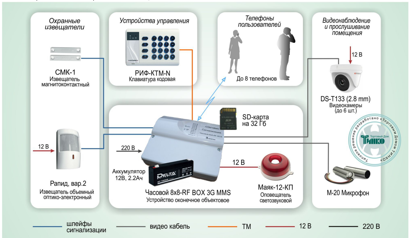
Схема построения системы охранной сигнализации на базе «Часовой 8x8 RF BOX 3G MMS»
