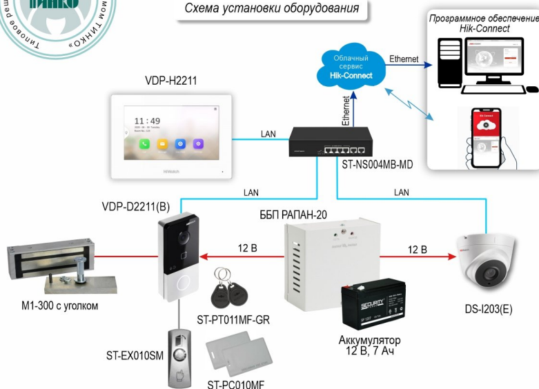
Схема установки оборудования
