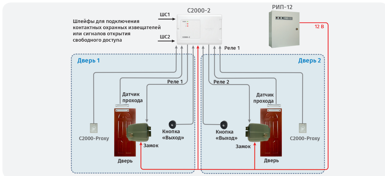
Рисунок 47. Режим работы «Две двери на вход»
