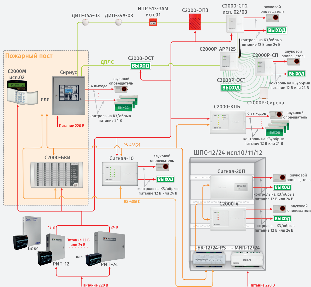
Рисунок 14. СОУЭ 1-го и 2-го типа на базе пульта «С2000М исп.02» и ППКУП «Сириус»
