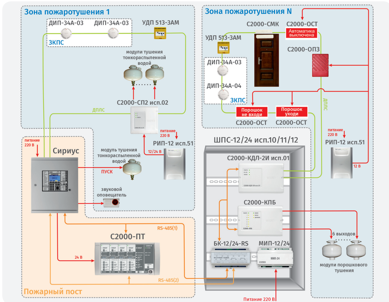
Рисунок 20. Реализация модульных установок порошкового и водяного тушения
