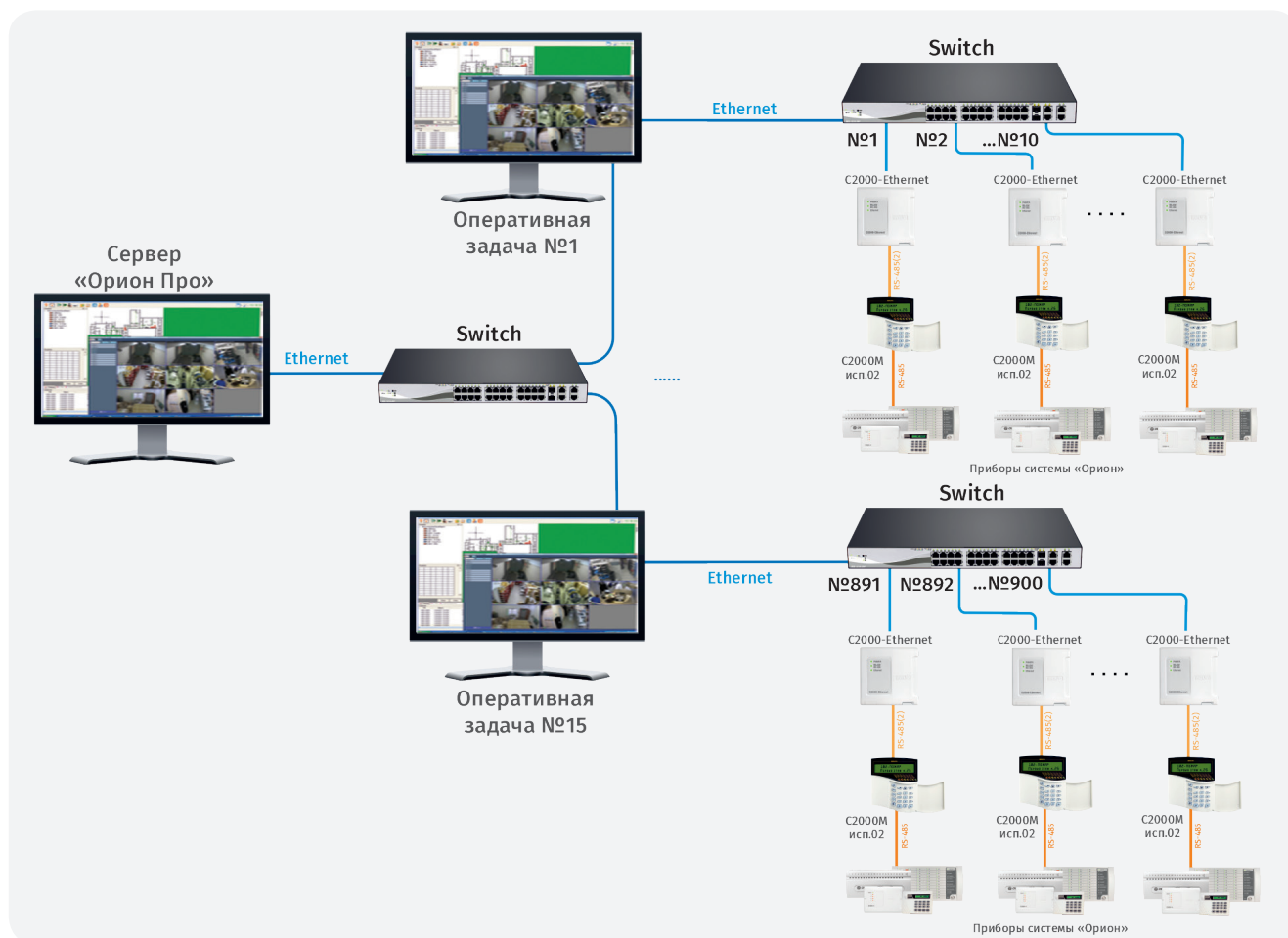
Рисунок 116. Пример построения системы с использованием «C2000-Ethernet» на 900 объектах
