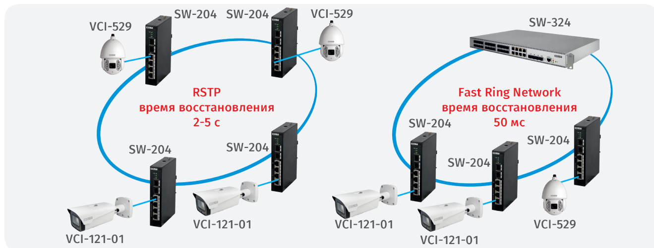
Рисунок 70. Примеры кольцевых топологий для построения периметральных систем видеонаблюдения
