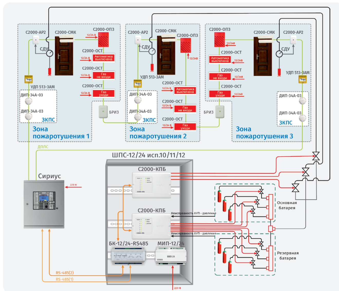
Рисунок 19. Реализация централизованных АУГПТ с резервной батареей
