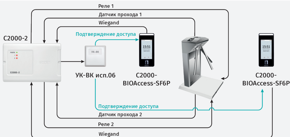
Рисунок 57. Использование C2000-BioAccess-SF6P в качестве биометрических считывателей
