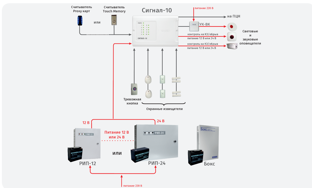
Рисунок 37. Автономное использование прибора «Сигнал-10»
