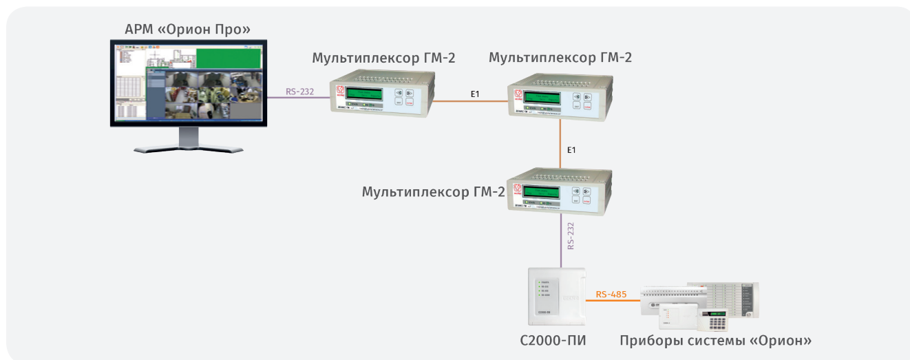
Рисунок 99. Структурная схема использования мультиплексора «ГМ-2» с АРМ «Орион»/«Орион Про» с подключением промежуточного мультиплексора (ремultipлексирование)
