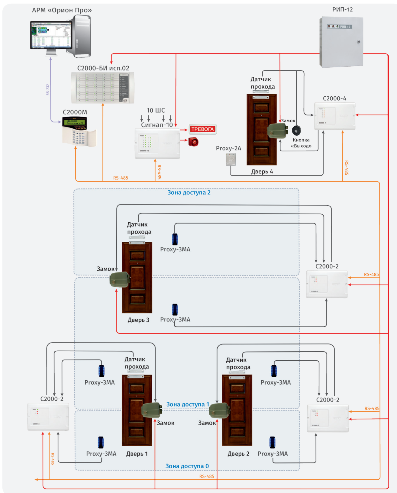
Рисунок 59. Сетевая СКУД с использованием программного обеспечения
