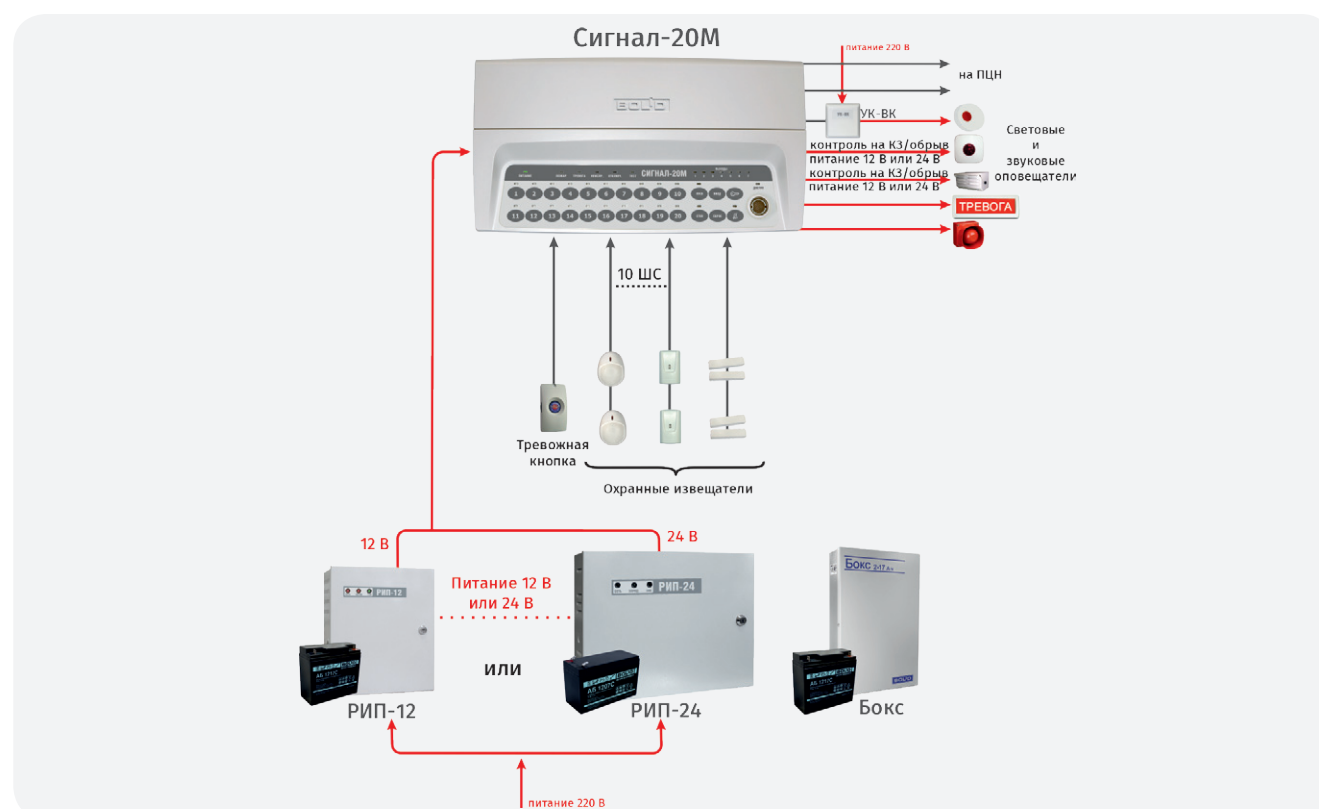
Рисунок 38. Автономное использование прибора «Сигнал-20М»
