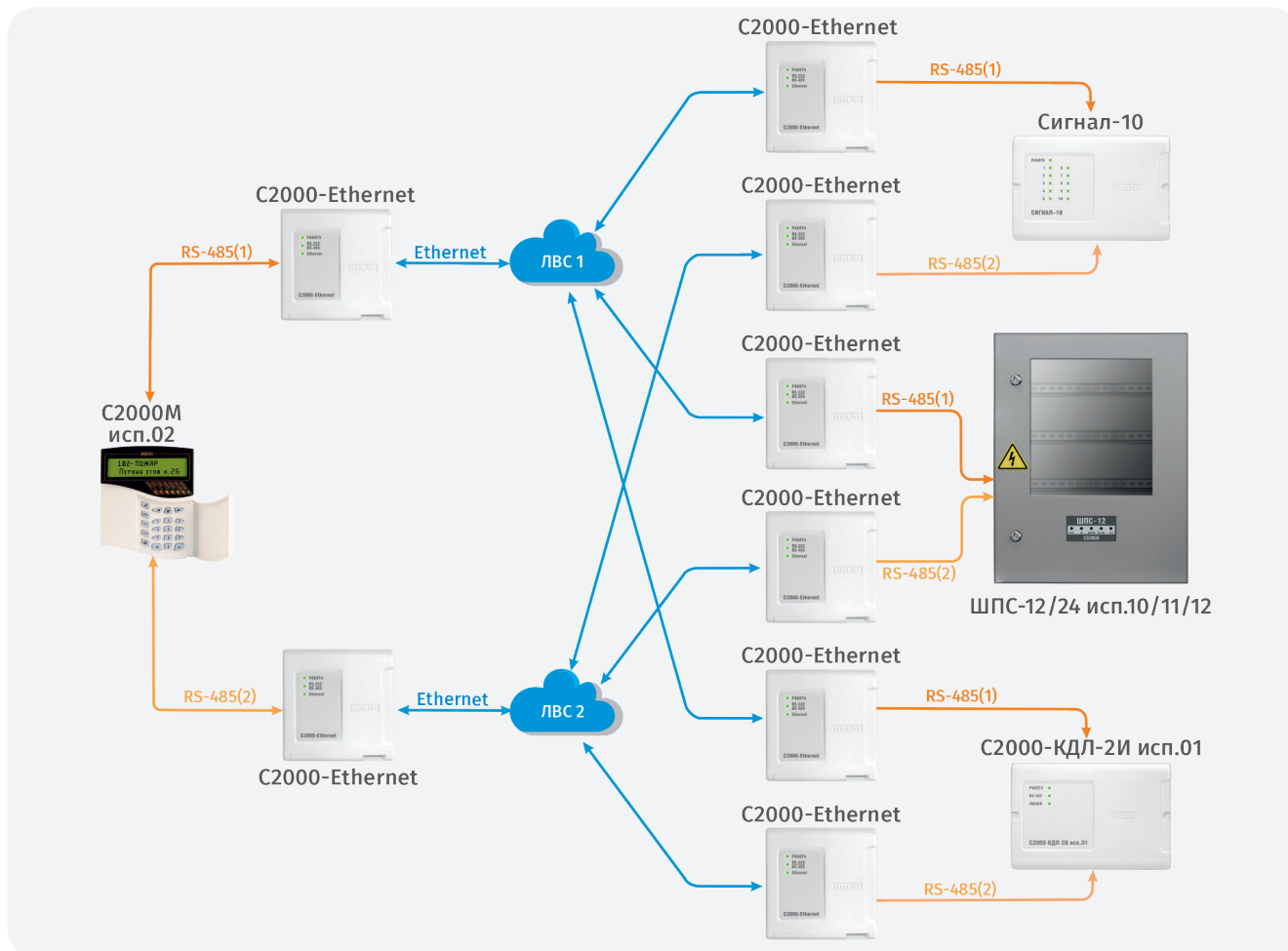
Рисунок 32. Передача резервированного RS-485 на пульт С2000М исп.02 по ЛВС
