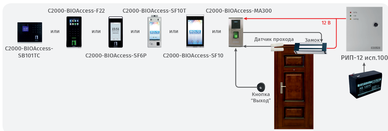
Рисунок 55. Биометрическая СКУД
