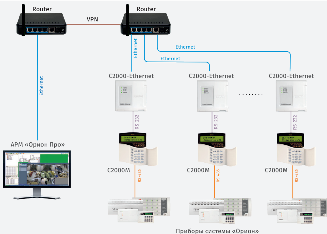
Рисунок 95. Пример использования «C2000-Ethernet» в глобальных сетях
