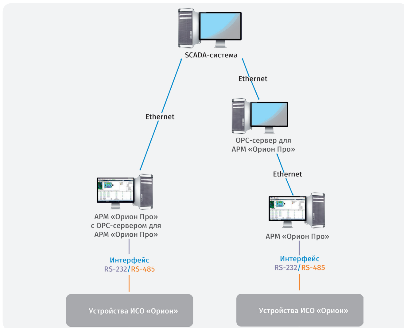
Рисунок 89. Передача данных в SCADA-систему
