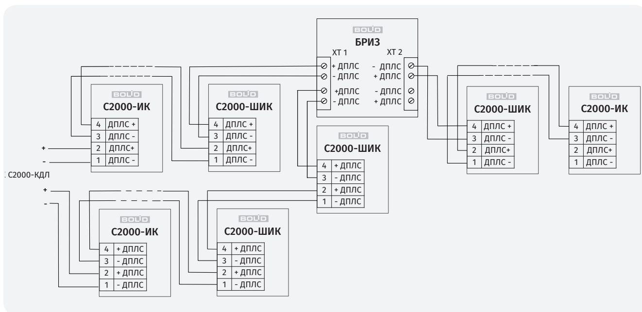
Рисунок 121. Схема подключения адресных извещателей в ДПЛС с топологией построения «кольцо»
