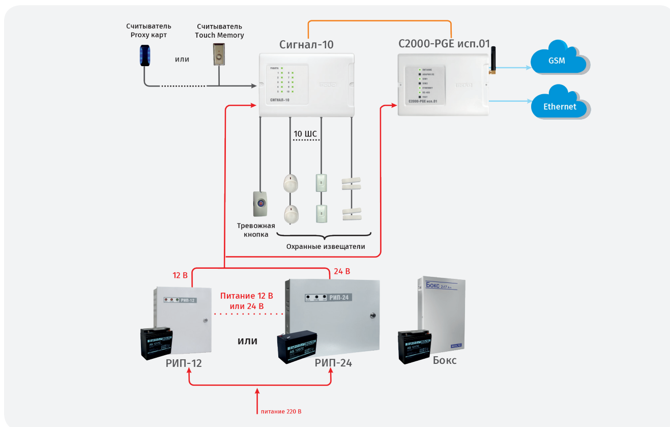
Рисунок 40. Система охранной сигнализации на базе прибора «Сигнал-10» и устройства «С2000-PGE исп.01»
