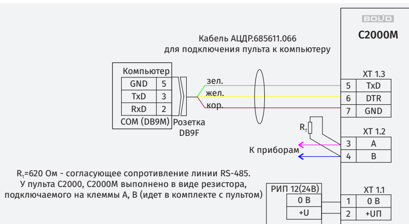
Рисунок 90. Схема подключения пульта «С2000М» к персональному компьютеру с АРМ «Орион Про»
