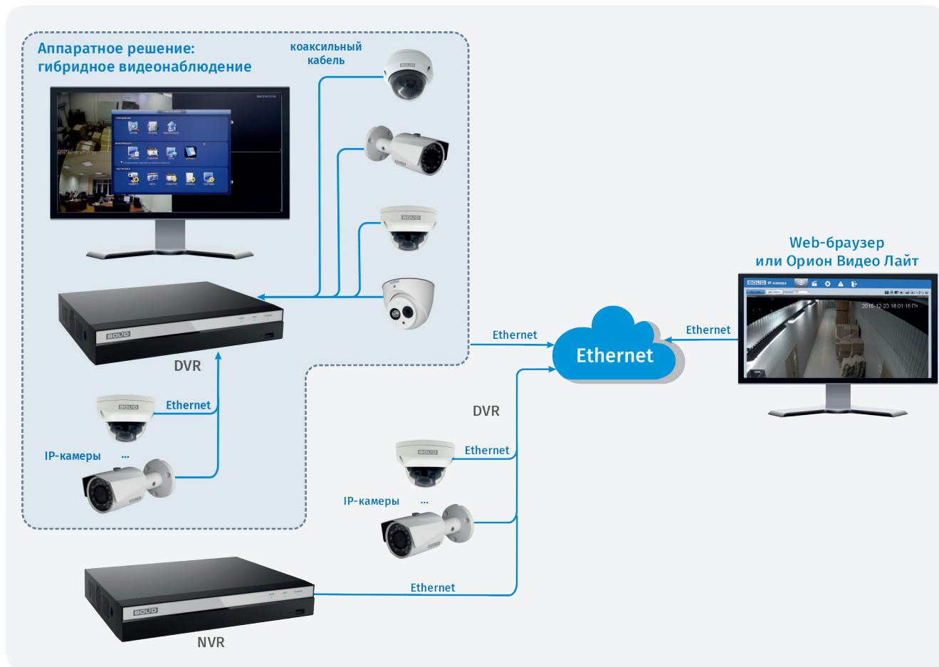
Рисунок 65. Локальная система видеонаблюдения на основе аппаратного решения
