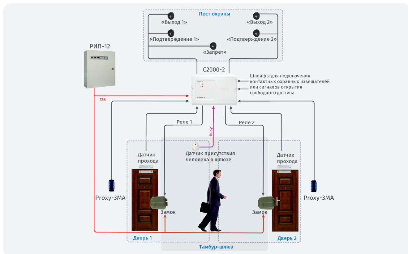
Рисунок 52. Режим работы «Шлюз»
