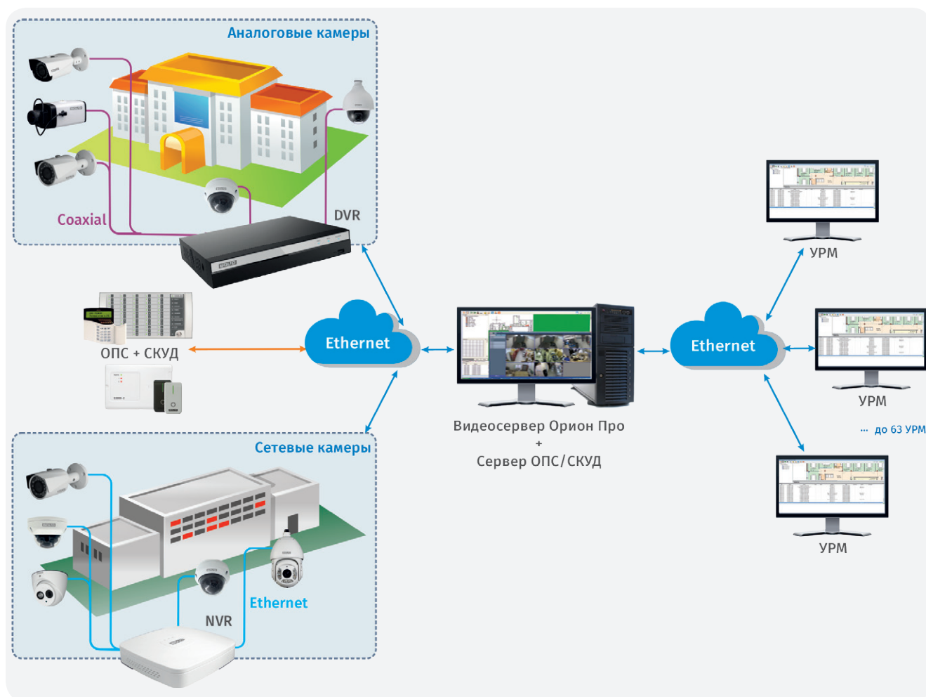
Рисунок 66. Сетевое видеонаблюдение напрямую с сетевых камер с удаленным рабочим местом на АРМ «Орион Про»
