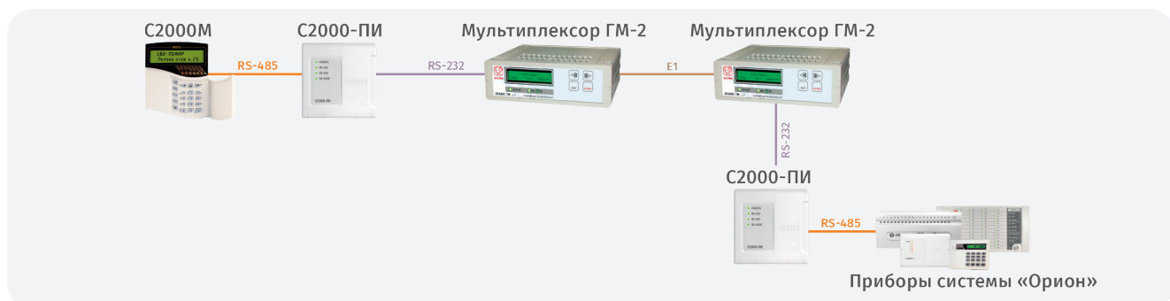
Рисунок 100. Структурная схема использования мультиплексора «ГМ-2» с пультом «C2000M»
