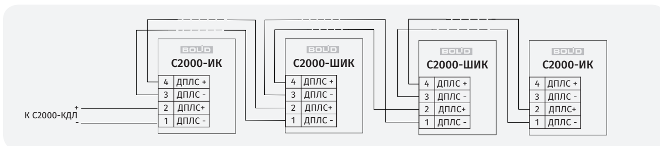
Рисунок 119. Схема подключения адресных извещателей в ДПЛС с топологией построения «шина»
