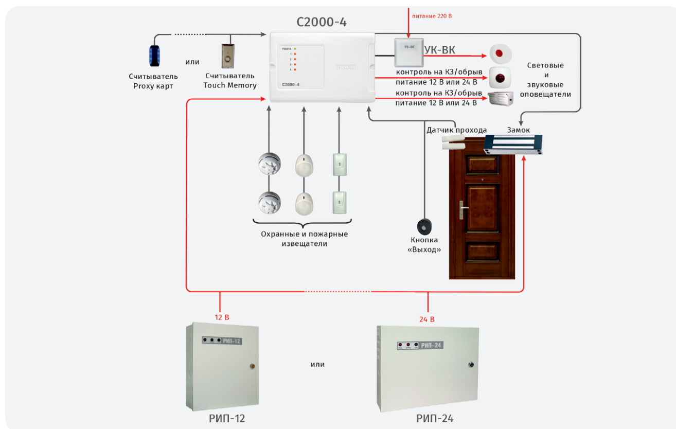
Рисунок 54. «С2000-4» с функционалом контроля доступа
