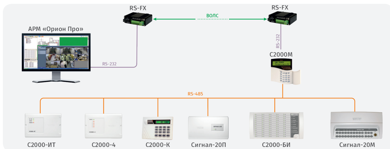
Рисунок 97. Типовая схема работы преобразователей RS-FX по протоколу «Орион Про»
