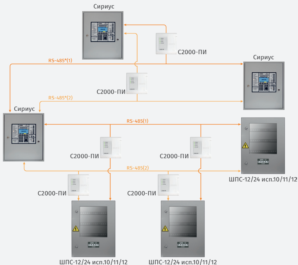
Рисунок 30. Структурная схема сети RS-485 с топологией «звезда» при помощи повторителей интерфейса
