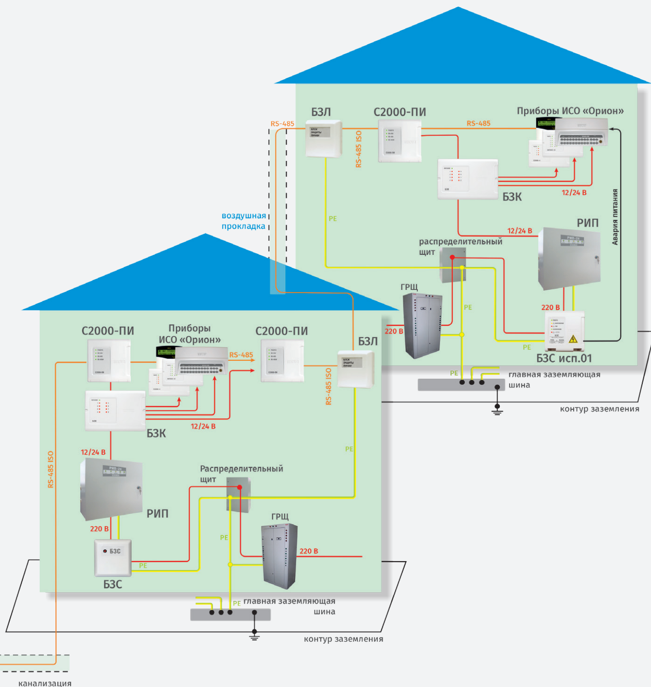
Рисунок 118. Схема подключения приборов с защитой интерфейса RS-485 от перенапряжений
