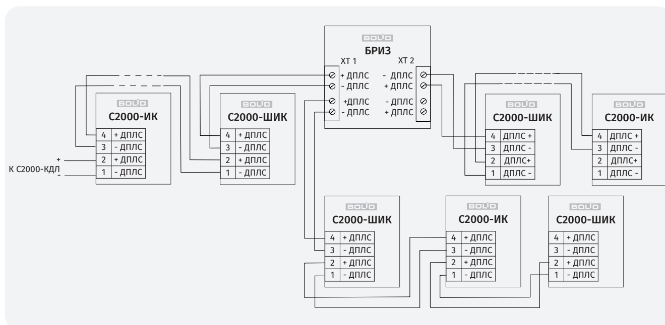
Рисунок 120. Схема подключения адресных устройств в ДПЛС с топологией построения «дерево»
