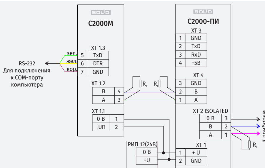
Рисунок 91. Схема подключения пультов «С2000М» к персональному компьютеру с АРМ «Орион Про» с гальванической изоляцией интерфейса RS-485
