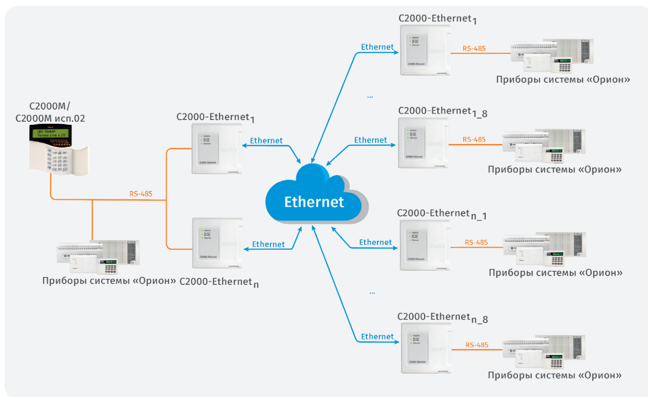
Рисунок 104. Структурная схема использования «C2000-Ethernet» с «C2000M»
