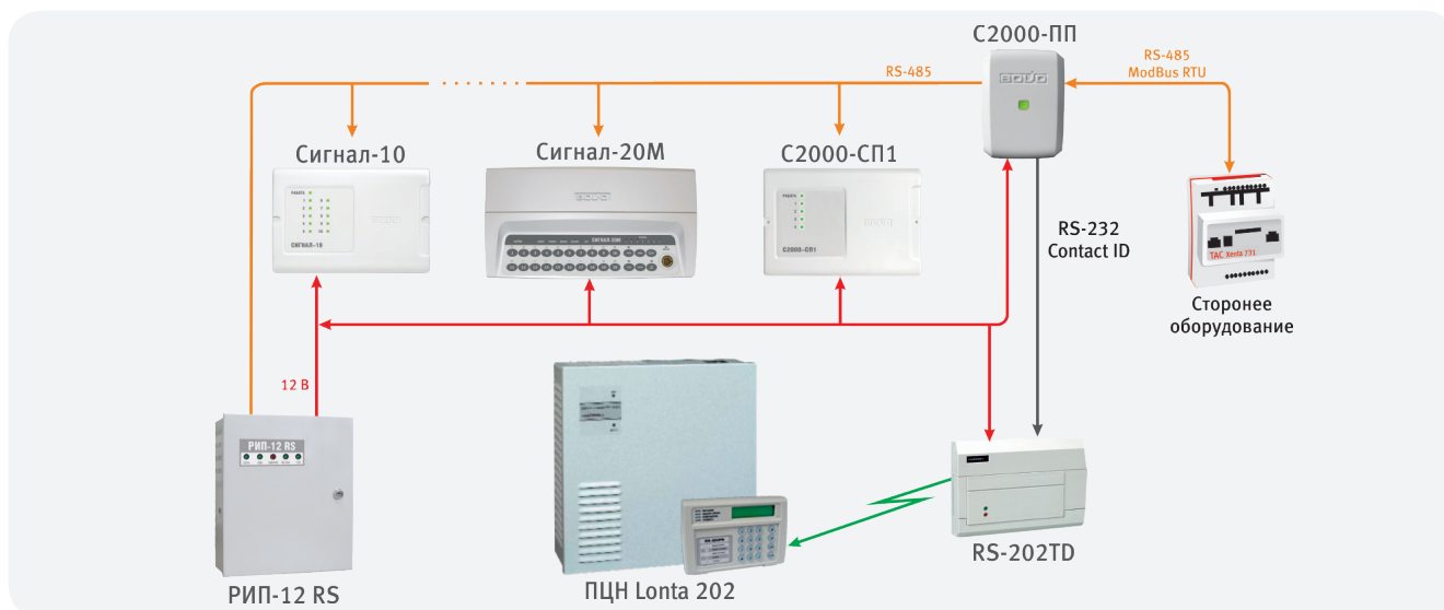
Рисунок 84. Применение «С2000-ПП» в ведущем режиме
