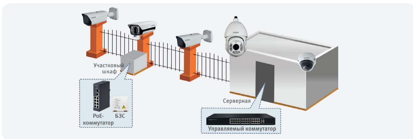
Рисунок 77. Типовые подходы к проектированию охраны протяженных периметров
