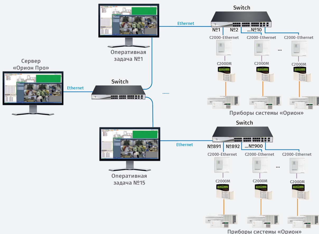
Рисунок 96. Пример построения системы с использованием «C2000-Ethernet» на 900 объектах
