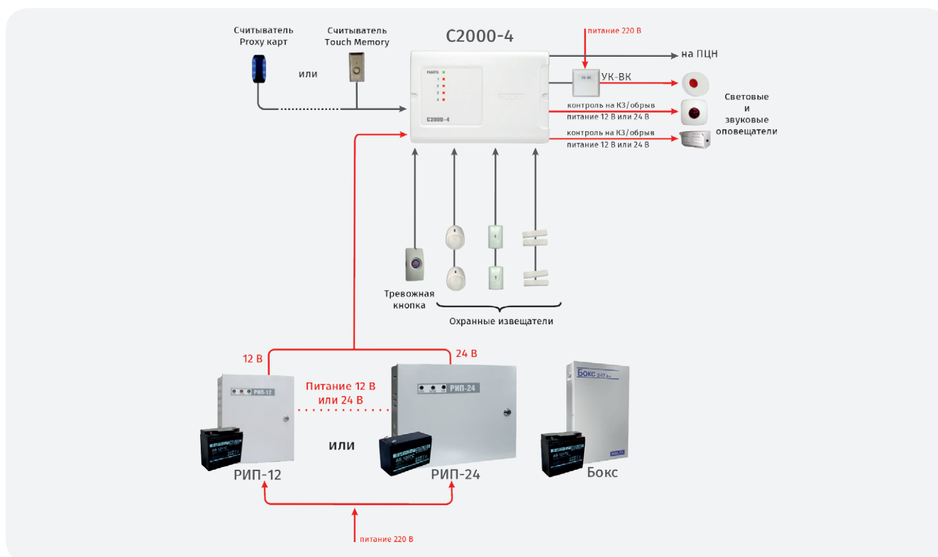
Рисунок 36. Автономное использование блока «С2000-4»
