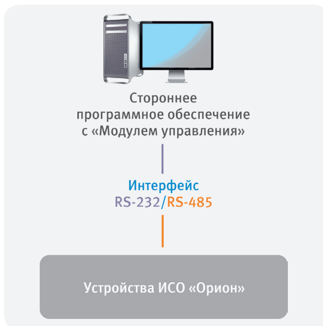
Рисунок 88. Интеграция с устройствами посредством «Модуля управления»
