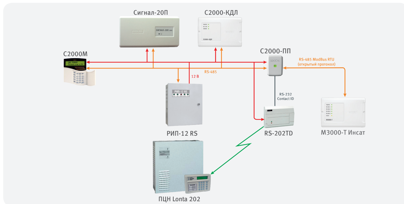
Рисунок 85. Применение «С2000-ПП» в ведомом режиме
