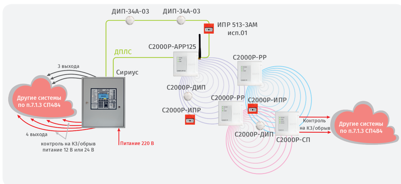
Рисунок 11. Радиоканальное расширение адресно-аналоговой системы пожарной сигнализации
