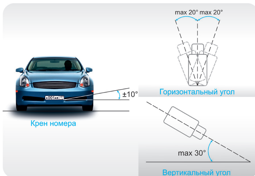
Рисунок 80. Видеонаблюдение с определением номеров на транспортном КПП
