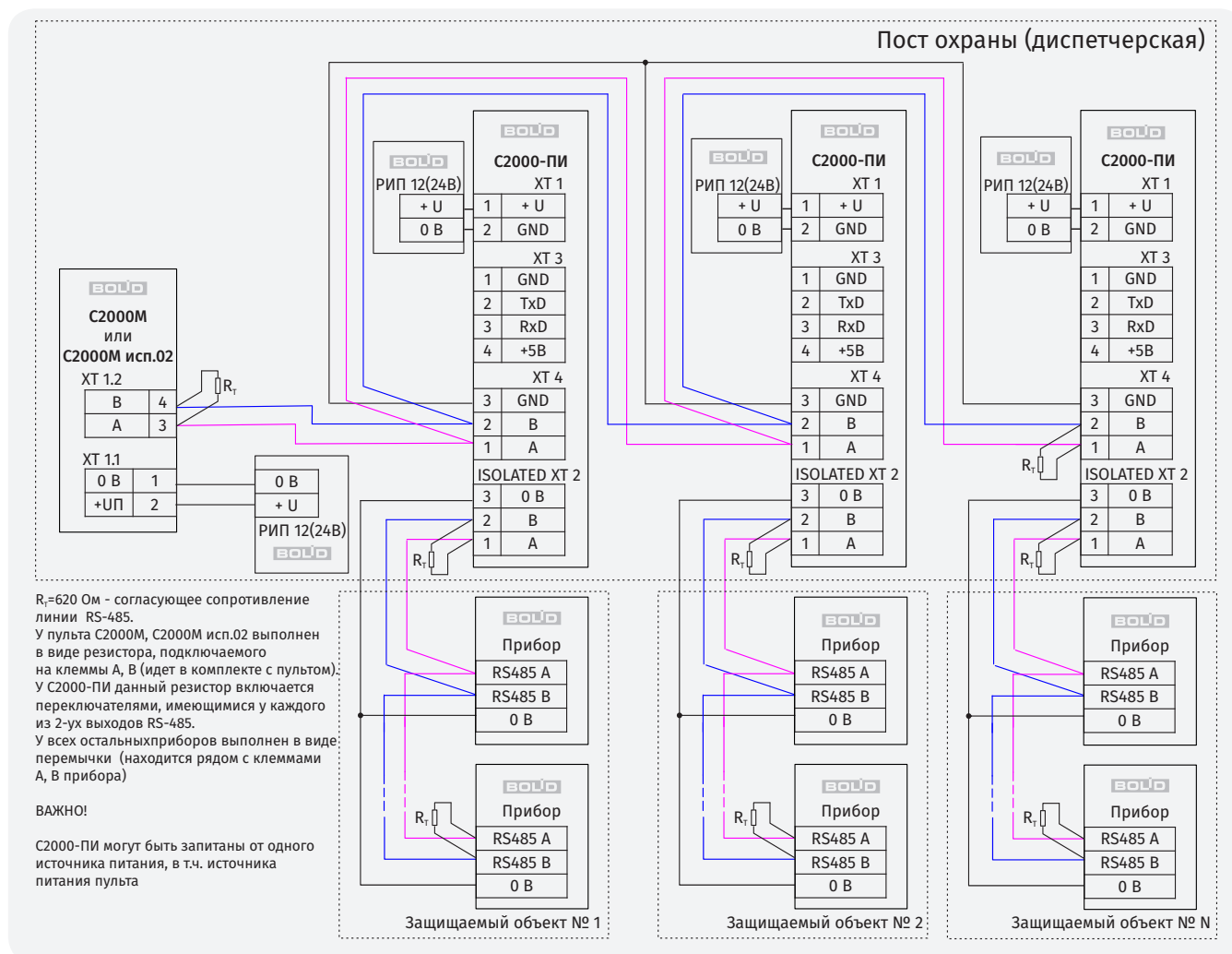
Рисунок 103. Построение сети RS-485 с топологией «звезда» при помощи повторителей
