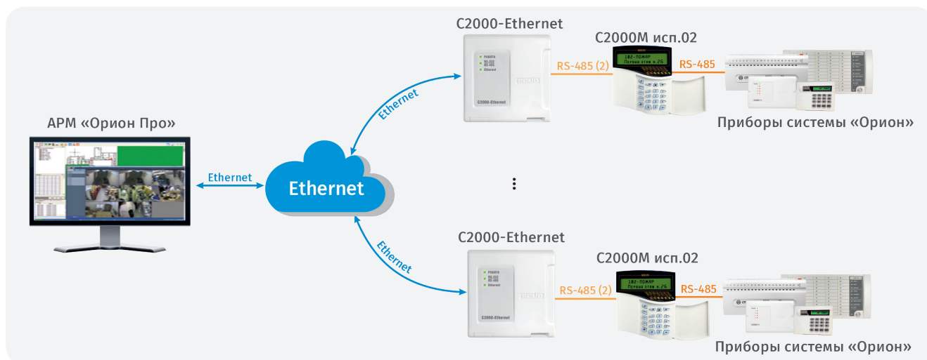
Рисунок 114. Типовая схема работы «С2000-Ethernet» по протоколу «Орион Про»
