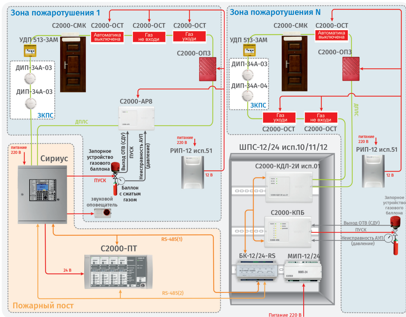
Рисунок 18. Реализация модульных АУГПТ
