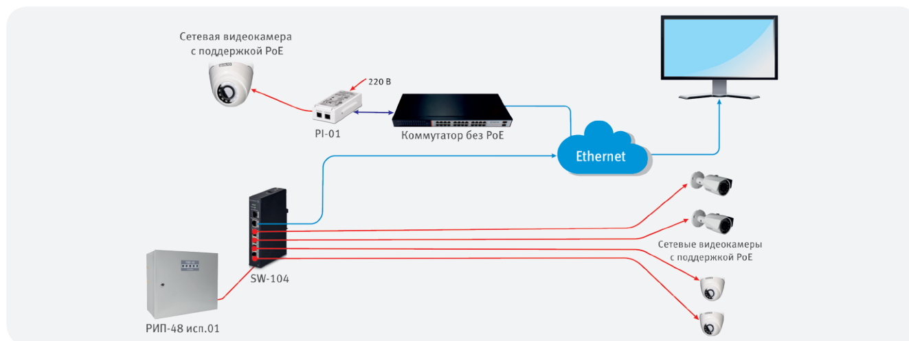
Рисунок 76. Организация электропитания сетевой системы видеонаблюдения с использованием технологии PoE
