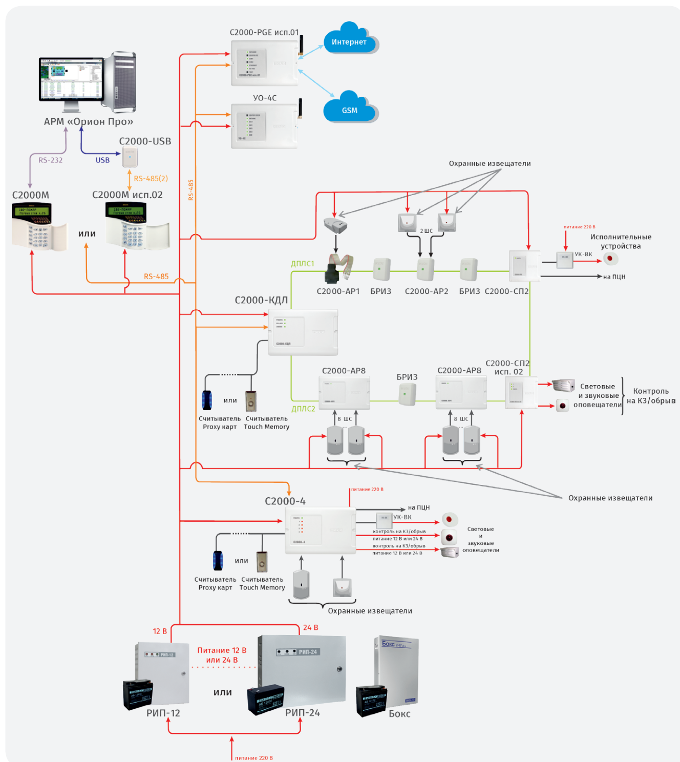
Рисунок 44. Комбинированная система охранной сигнализации
