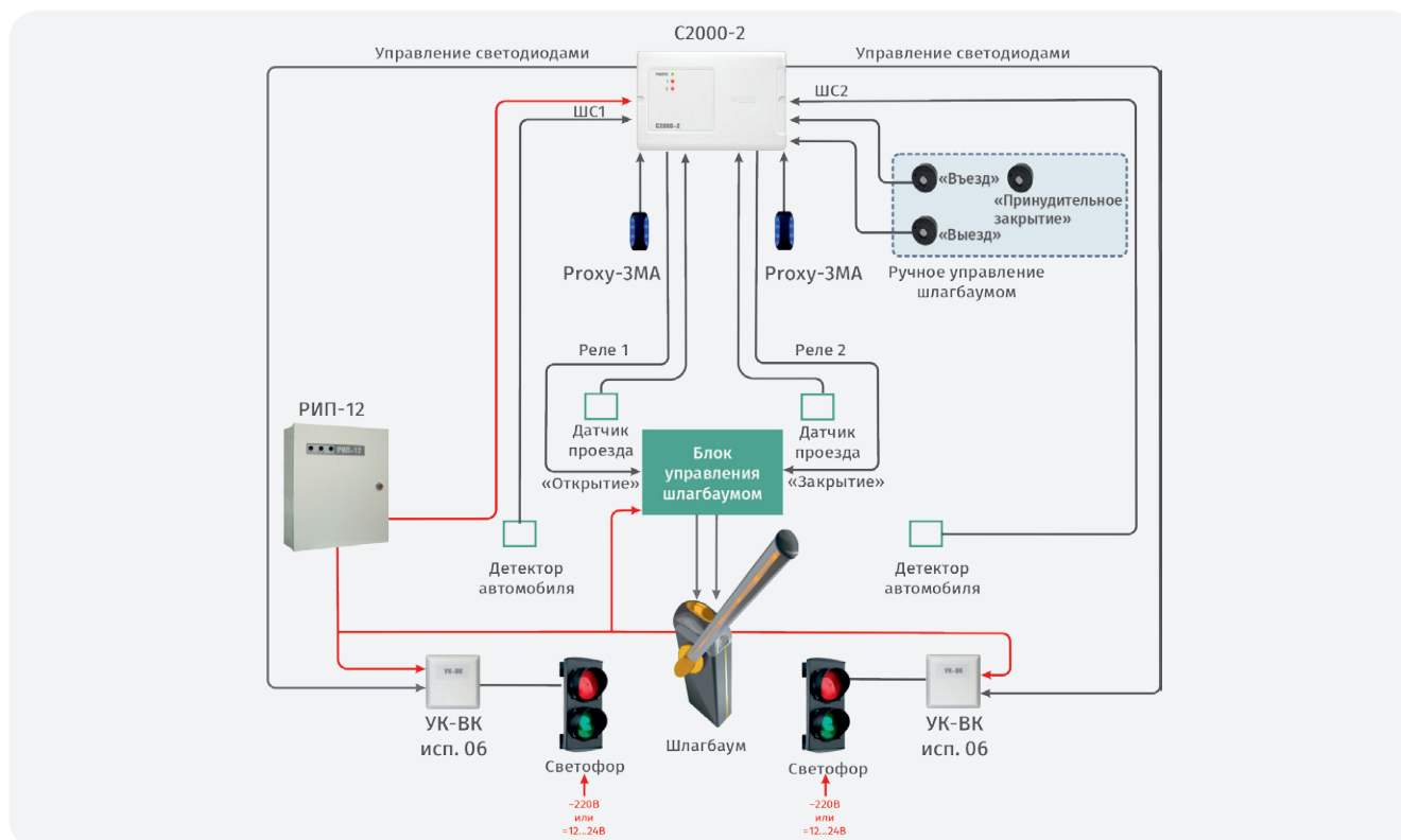
Рисунок 51. Режим работы «Шлагбаум»
