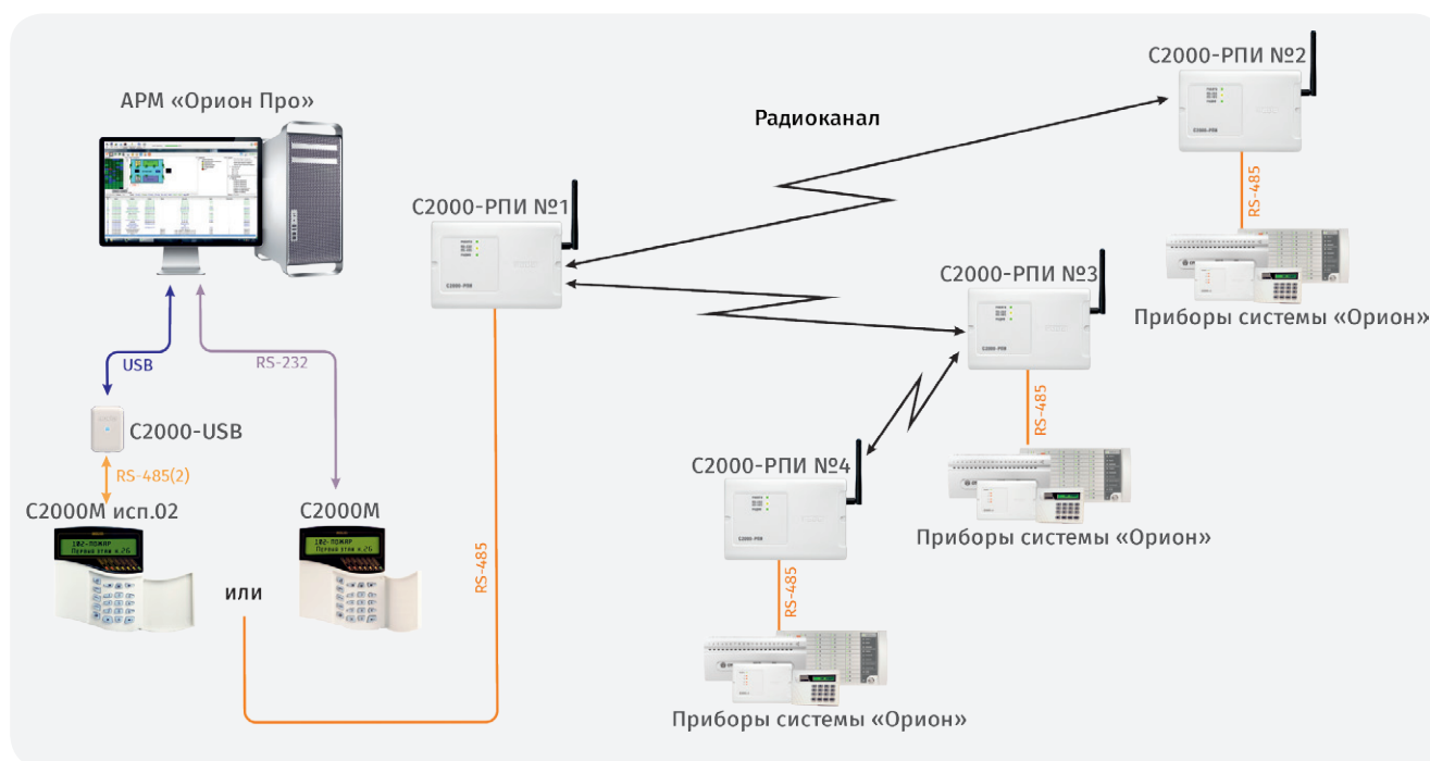
Рисунок 108. Структурная схема использования «C2000-РПИ» с АРМ «Орион Про» и «C2000М»/ «C2000М исп.02», соединение «точка-многоточка» с ретрансляцией
