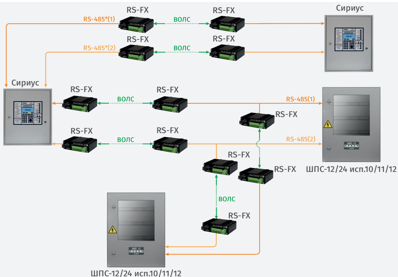
Рисунок 31. Структурная схема использования преобразователей RS-FX
