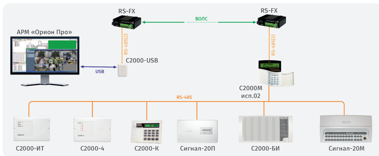
Рисунок 117. Типовая схема работы преобразователей RS-FX по протоколу «Орион Про»
