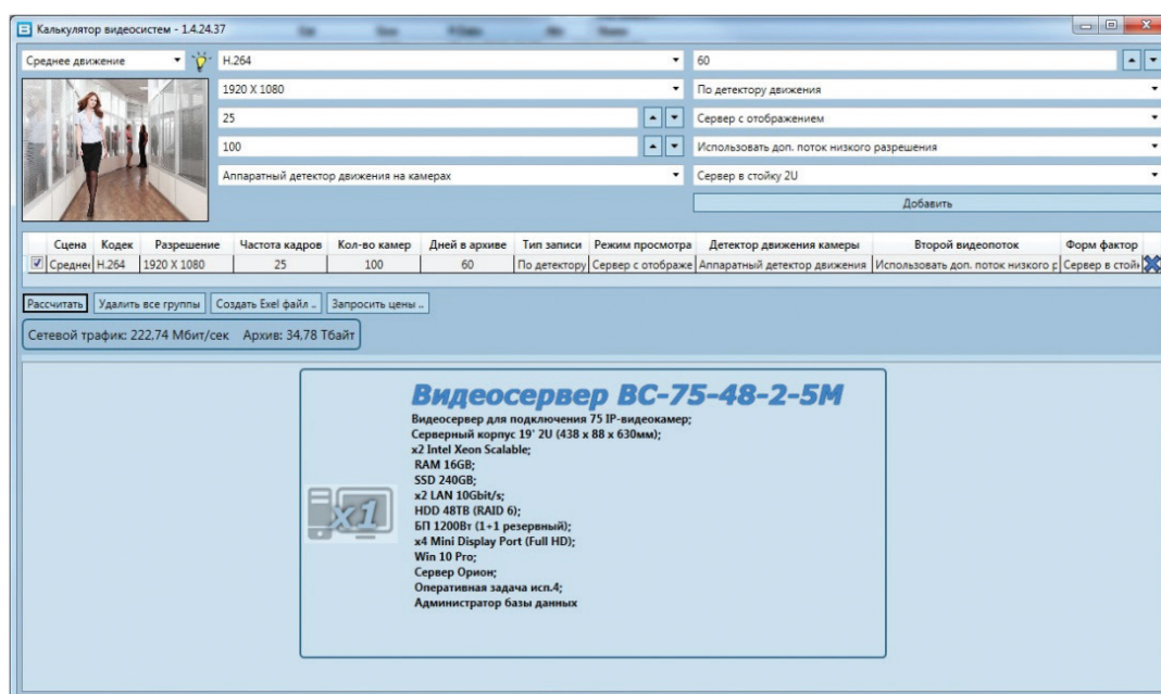
Рисунок 72. Пример рабочего интерфейса утилиты «Калькулятор видеосистемы» производства компании Бolid
