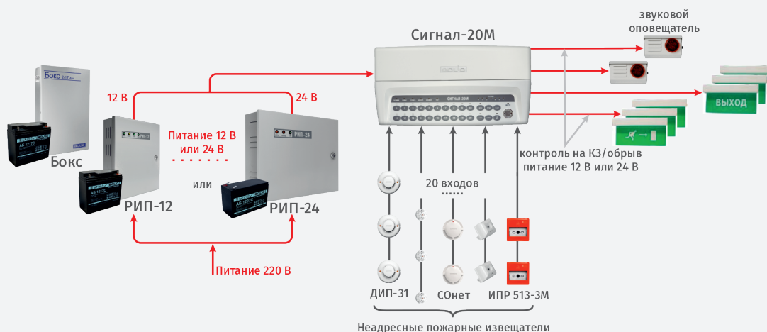
Рисунок 13. СОУЭ 1-го и 2-го типа на базе ППКУП «Сигнал-20М»
