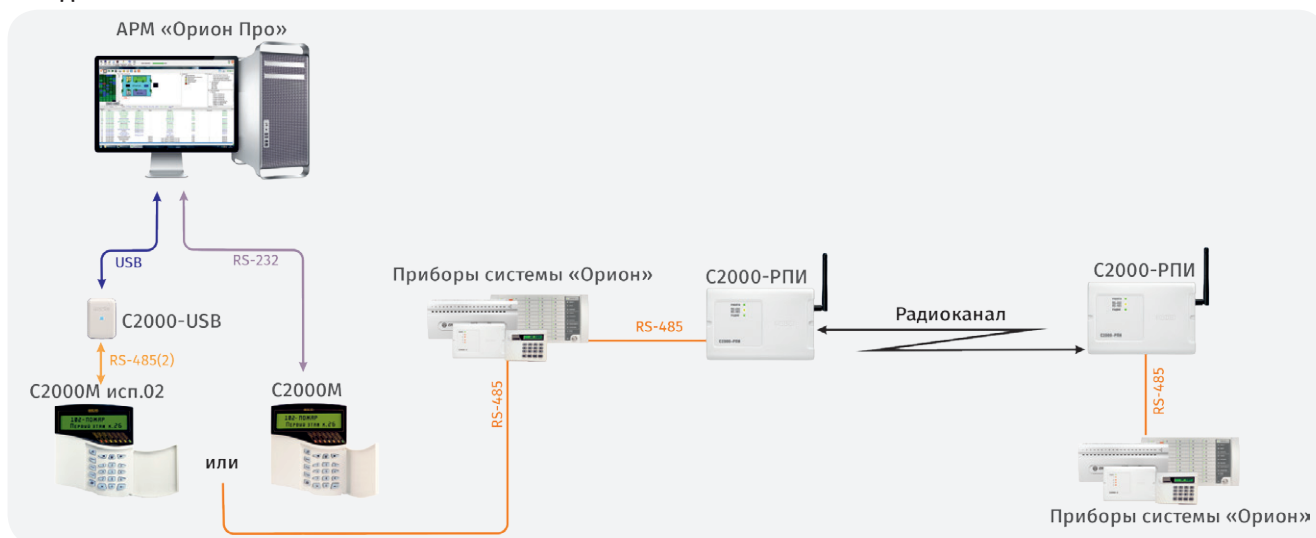
Рисунок 106. Структурная схема использования «С2000-РПИ» с АРМ «Орион Про» и «С2000М»/ «С2000М исп.02», соединение «точка-точка»
