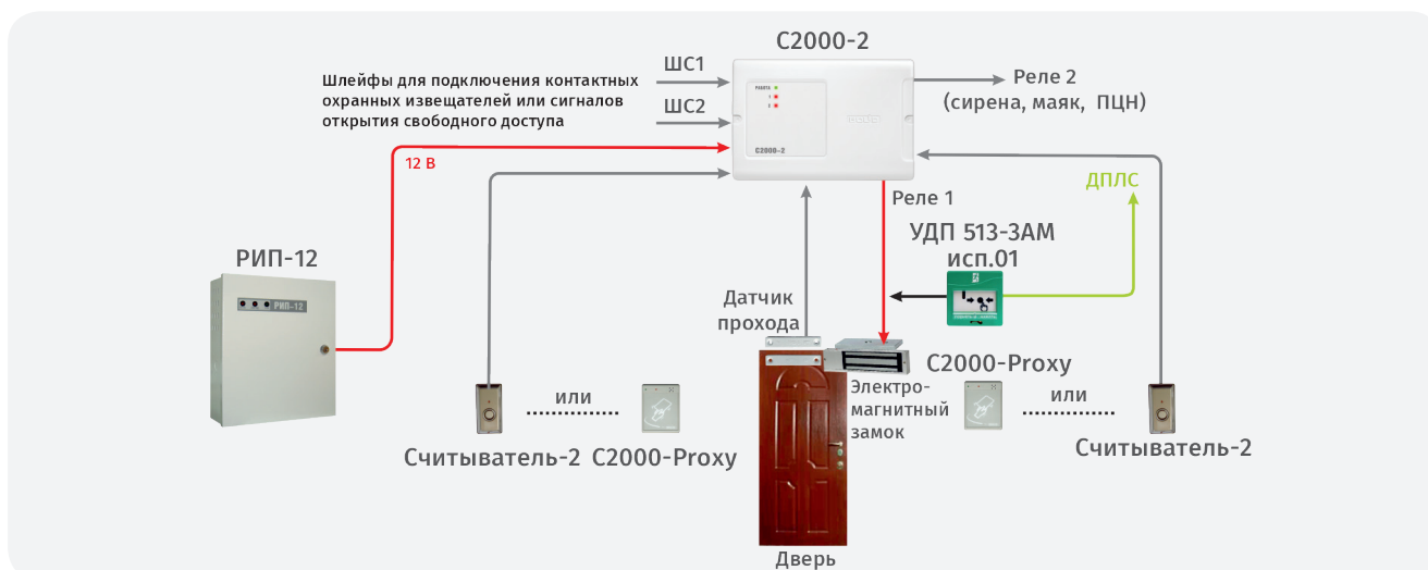
Рисунок 48. Режим работы «Одна дверь на вход/выход»
