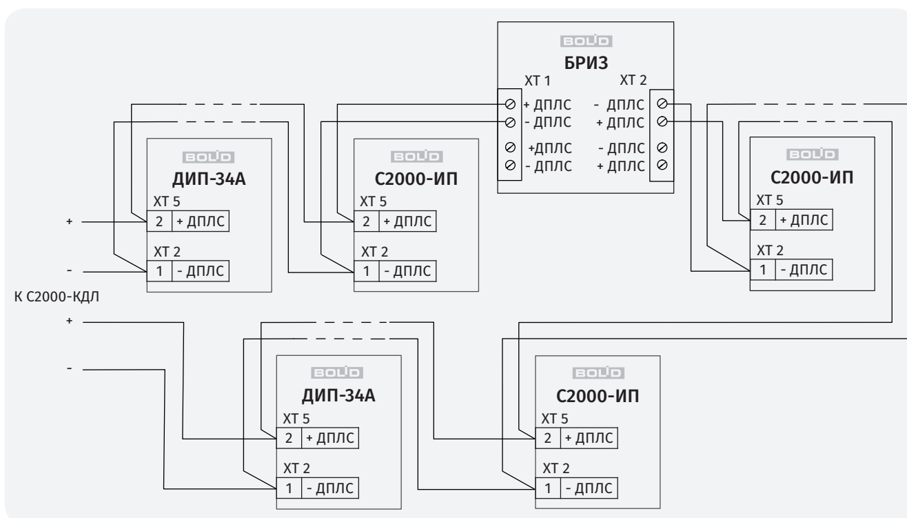
Рисунок 34. Схема подключения адресных извещателей в ДПЛС с топологией «кольцо»
