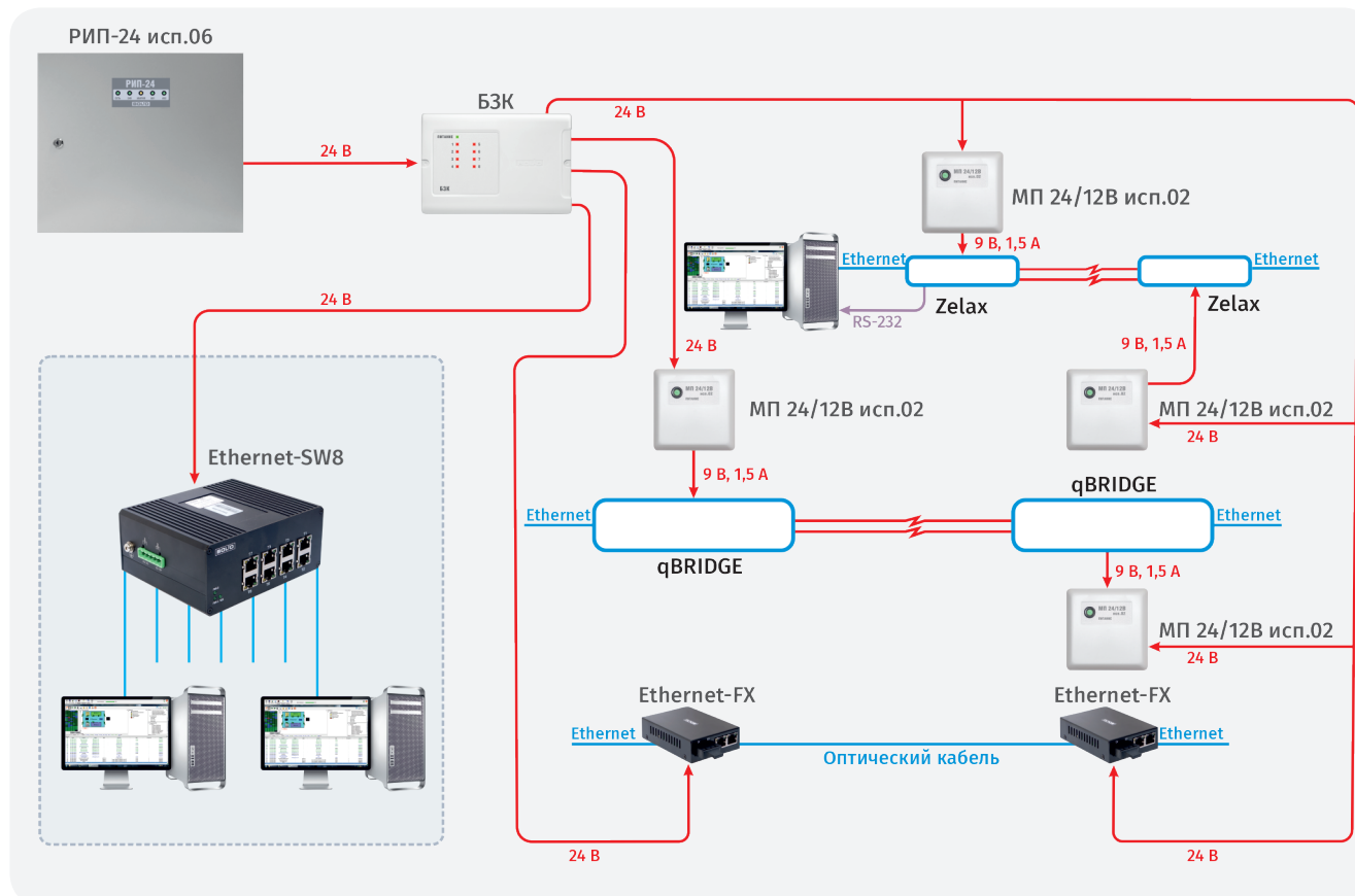
Рисунок 62. Электропитание сетевого каналообразующего оборудования
