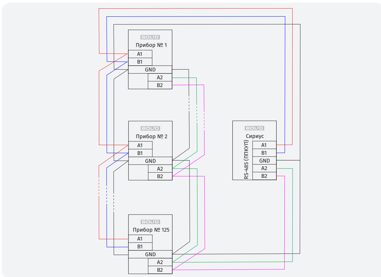
Рисунок 29. Структурная схема резервированного RS-485 интерфейса с топологией «кольцо»
