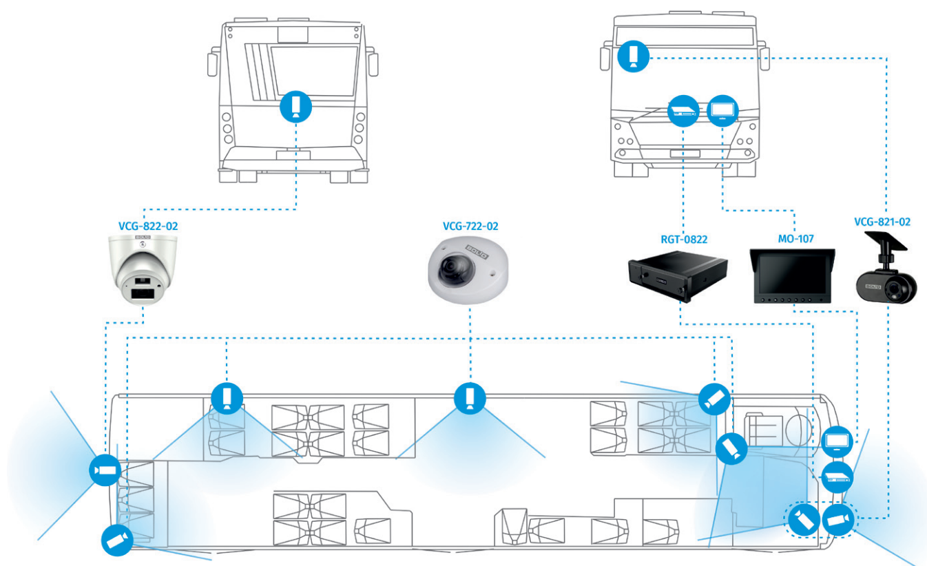
Рисунок 79. Схема расположения комплекса видеонаблюдения для транспортных средств
