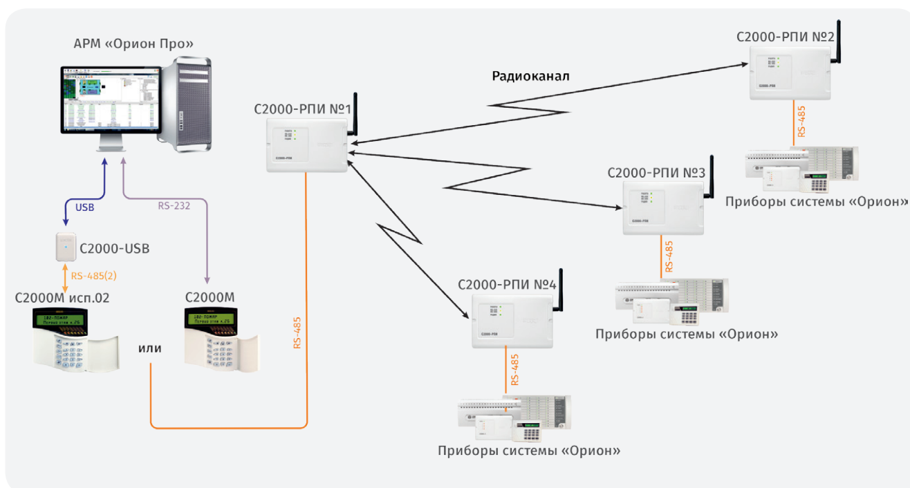
Рисунок 107. Структурная схема использования «С2000-РПИ» с АРМ «Орион Про» и «С2000М»/ «С2000М исп.02», соединение «точка-многоточка»
