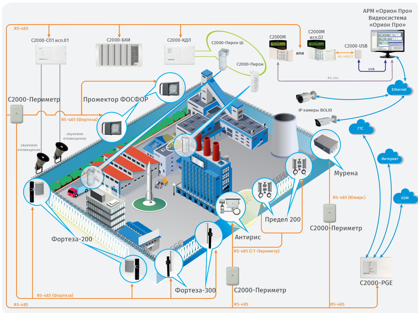
Рисунок 45. Система охраны периметра
