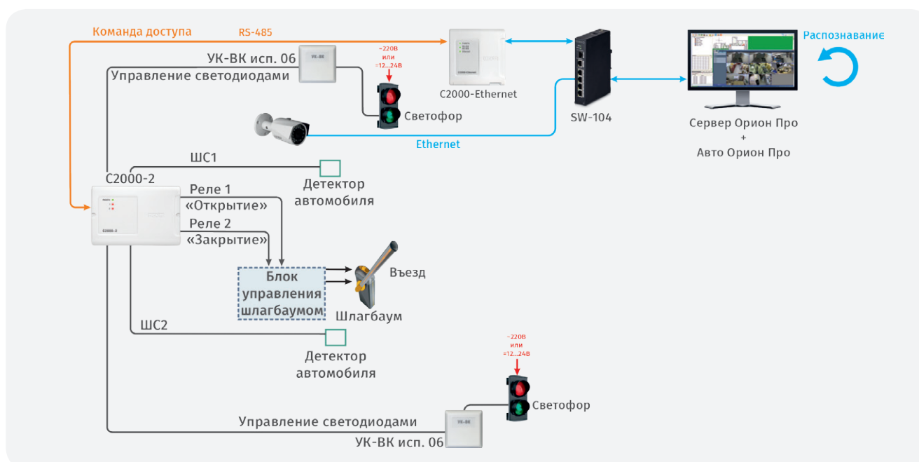
Рисунок 81. Видеонаблюдение с определением номеров на транспортном КПП
