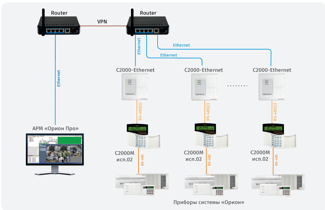
Рисунок 115. Пример использования «С2000-Ethernet» в глобальных сетях
