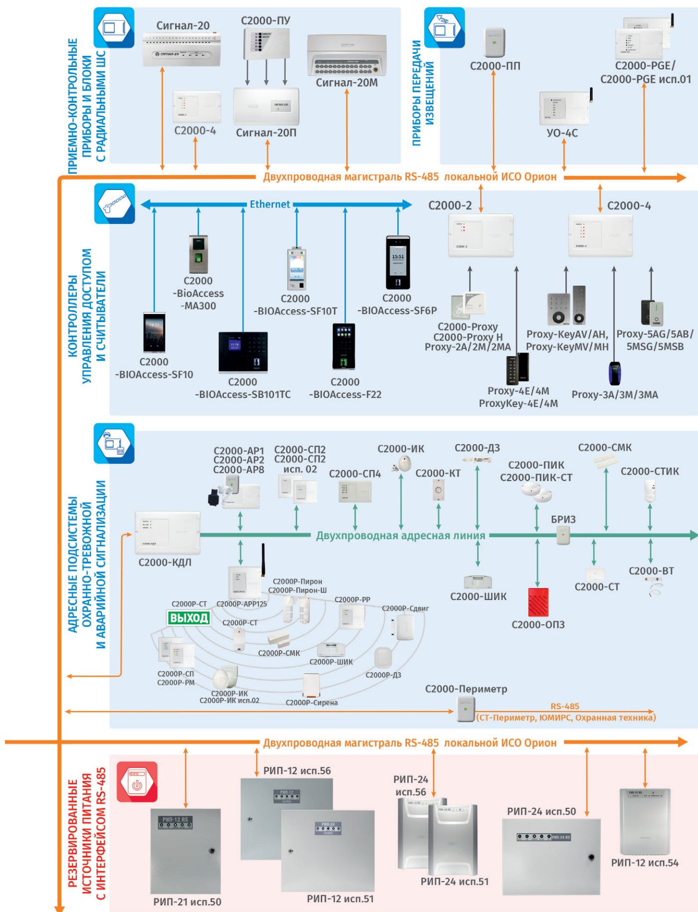
Рисунок 35. Структурная схема систем охраны и безопасности ИСО «Орион»
