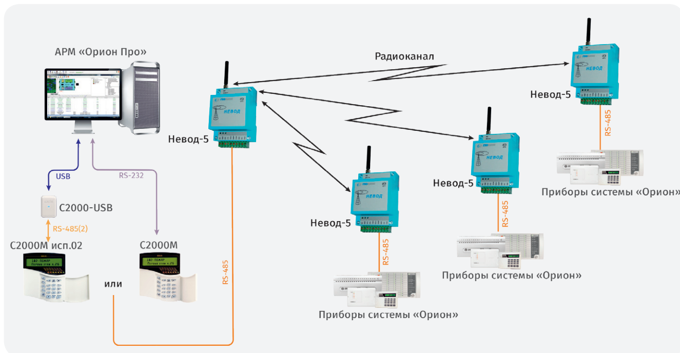
Рисунок 109. Структурная схема использования «Невод-5» с АРМ «Орион Про» и «С2000М»/ «С2000М исп.02», соединение «точка-многоточка»
