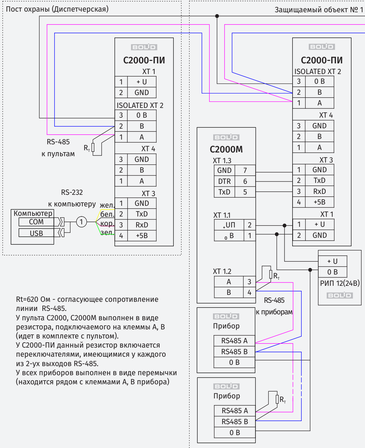
Рисунок 93. Схема подключения нескольких пультов
