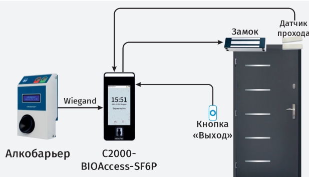
Рисунок 56. Подключение алкотестеров к биометрическим контроллерам
