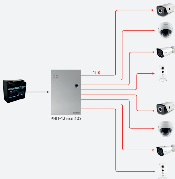
Рисунок 74. Организация питания видеокамер с помощью многоканального источника резервированного питания РИП-12 исп.108
