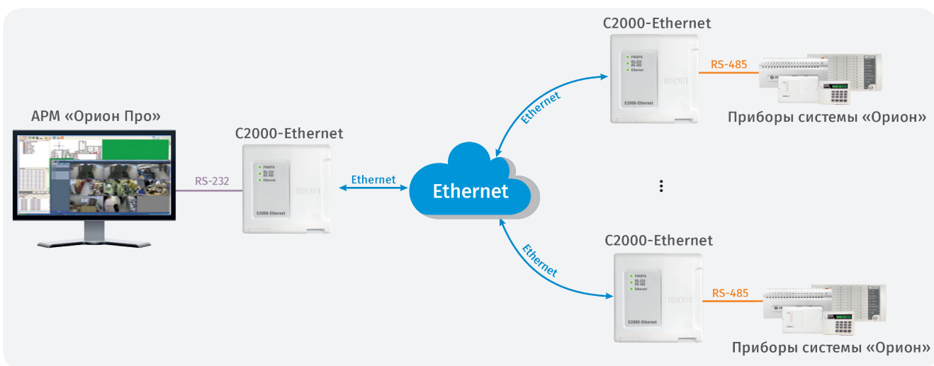
Рисунок 111. Типовая схема работы «С2000-Ethernet» по протоколу «Орион»
