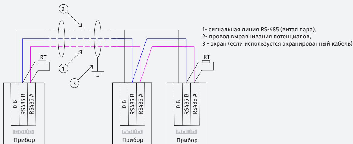
Рисунок 101. Схема подключения приборов к магистральному интерфейсу RS-485
