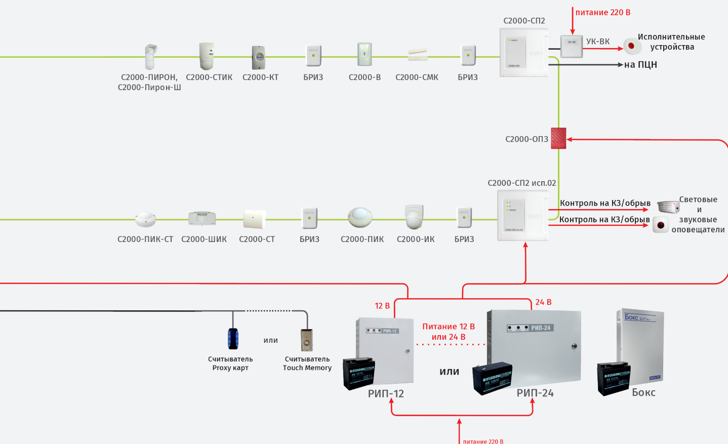
Рисунок 42. Адресная система охранной сигнализации
