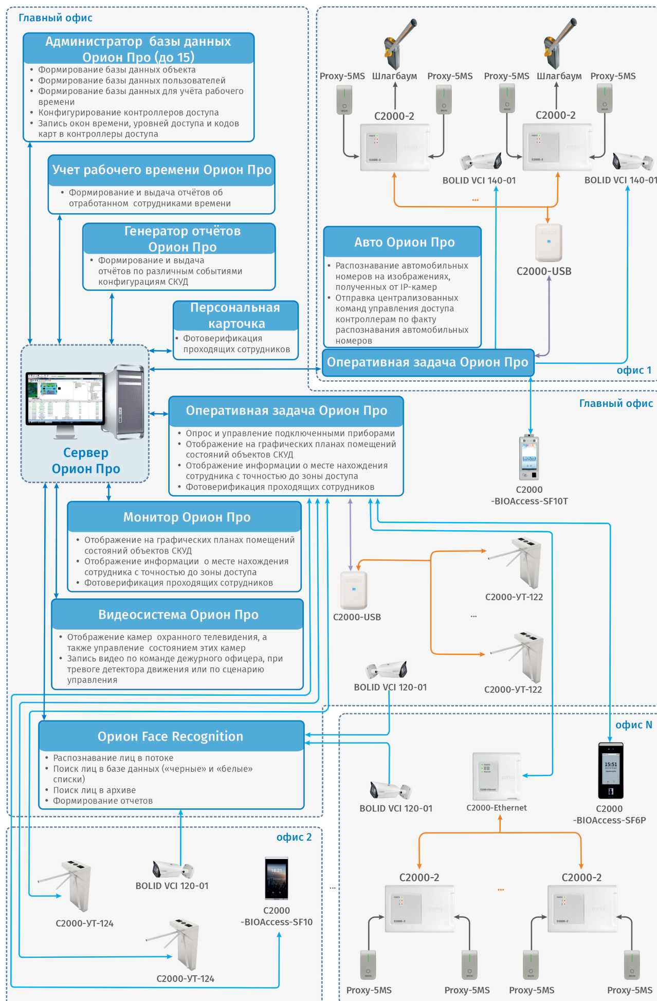
Рисунок 60. Системы контроля доступа с программным обеспечением
