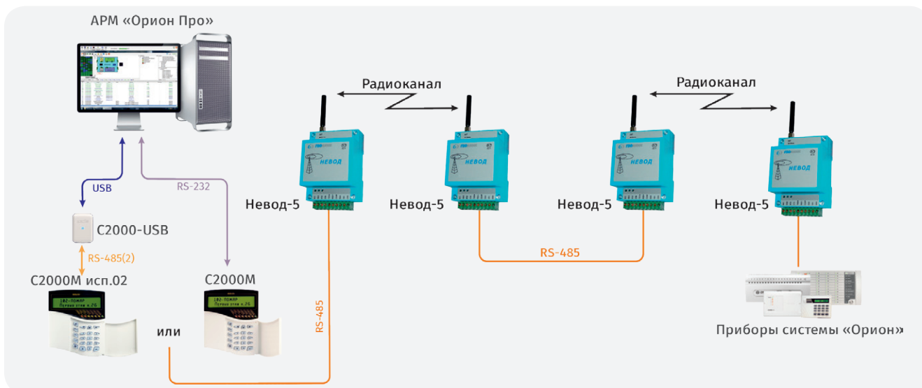
Рисунок 110. Структурная схема использования «Невод-5» с АРМ «Орион Про» и «С2000М»/«С2000М исп.02», соединение «точка-точка» с ретрансляцией
