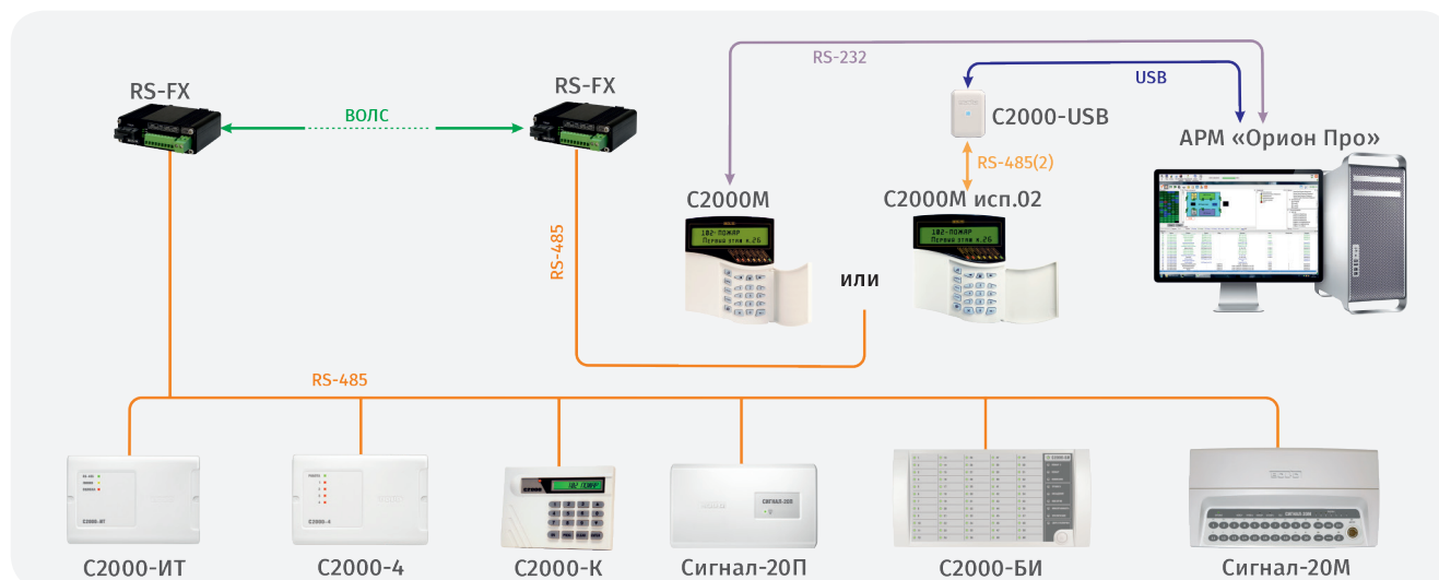
Рисунок 105. Структурная схема использования преобразователей RS-FX с АРМ «Орион Про» и «С2000М»/ «С2000М исп.02»
