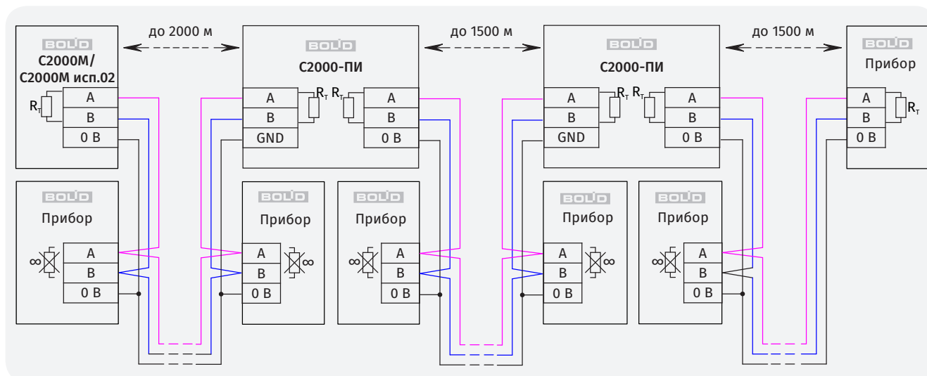
Рисунок 102. Увеличение длины линии RS-485 с помощью повторителей интерфейса
