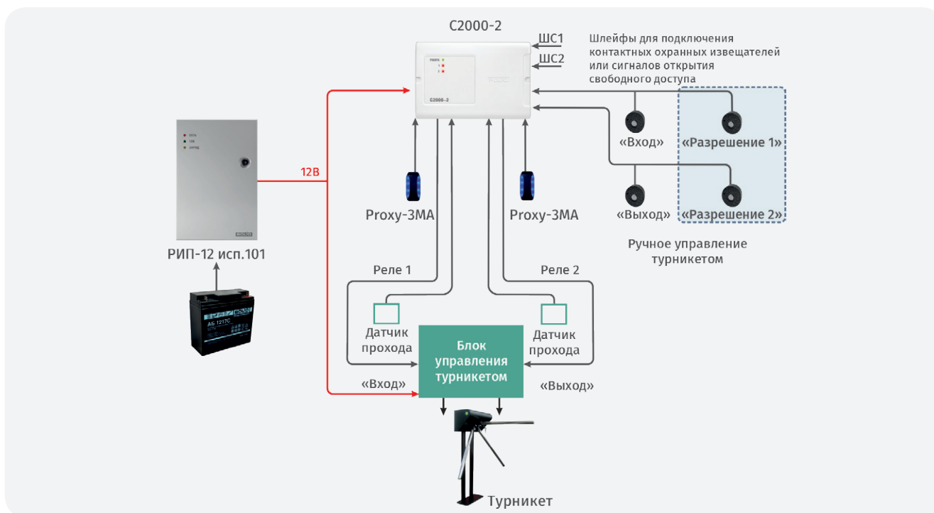
Рисунок 49. Режим работы «Турникет»
