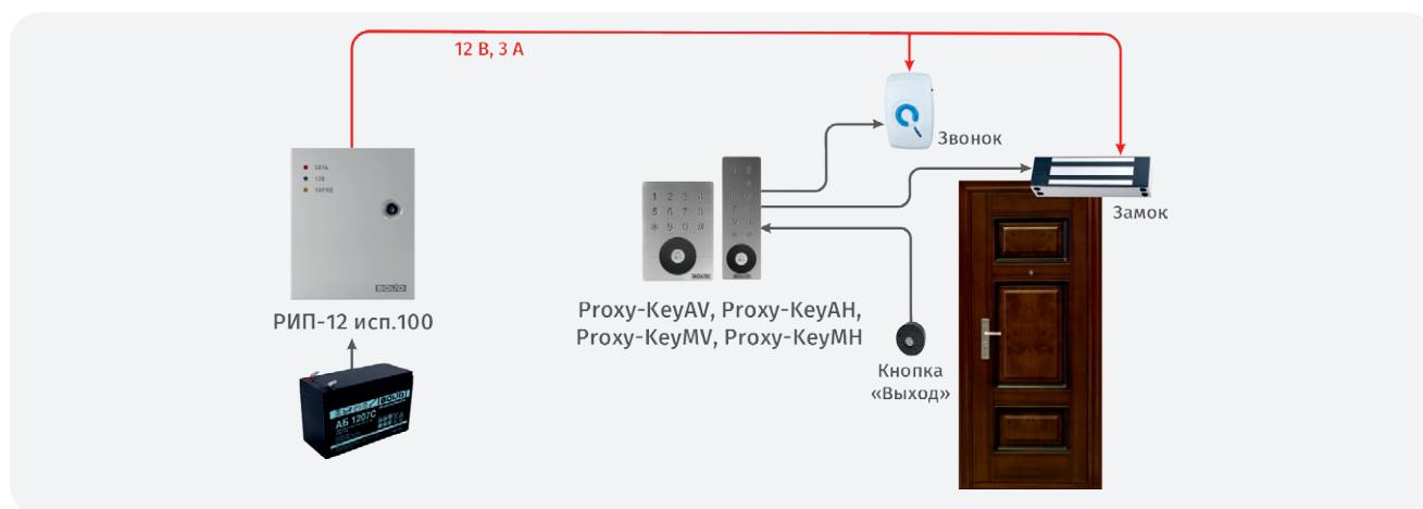
Рисунок 58. «Proxy-KeyAV/AH», «Proxy-KeyMV/MH»
