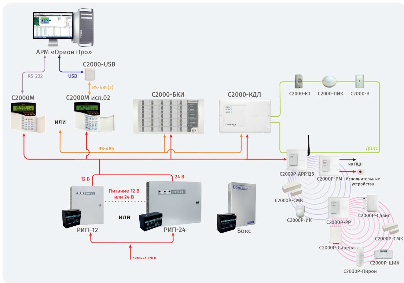
Рисунок 43. Адресная радиоканальная система на основе «C2000P-APP125»
