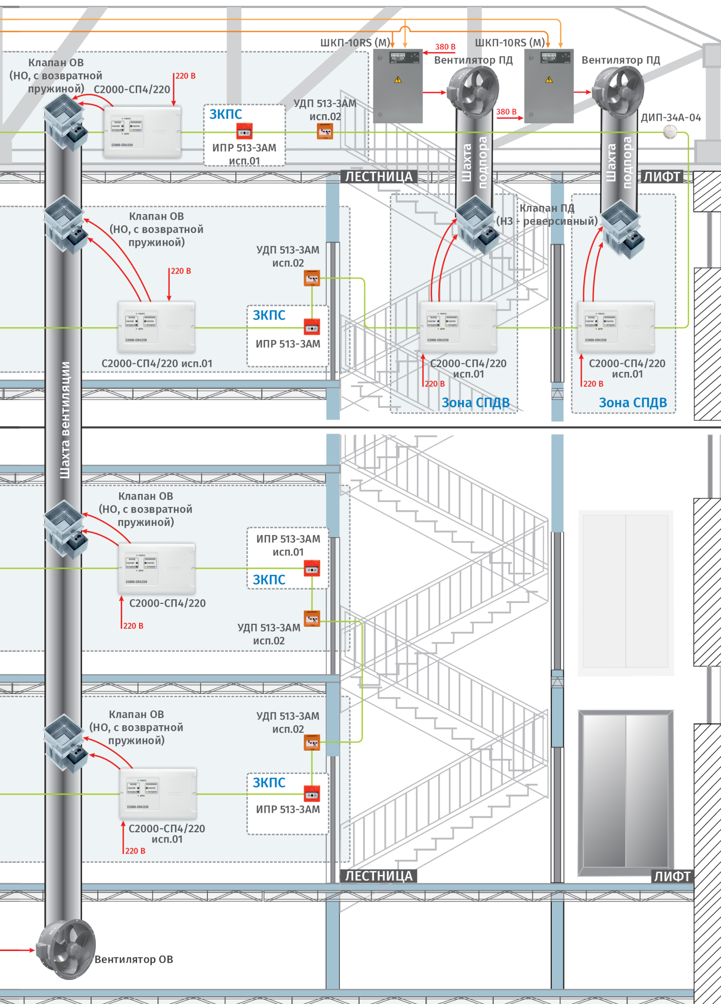
Рисунок 17. СПДВ в ИСО «Орион»
