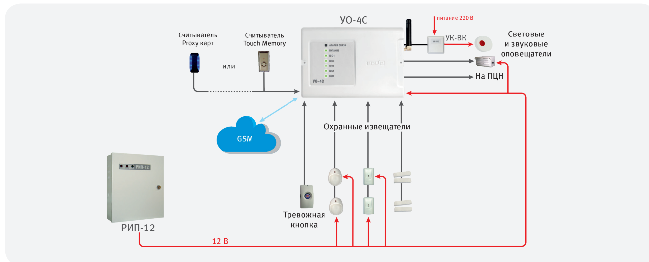
Рисунок 39. Автономное использование «YO-4C»
