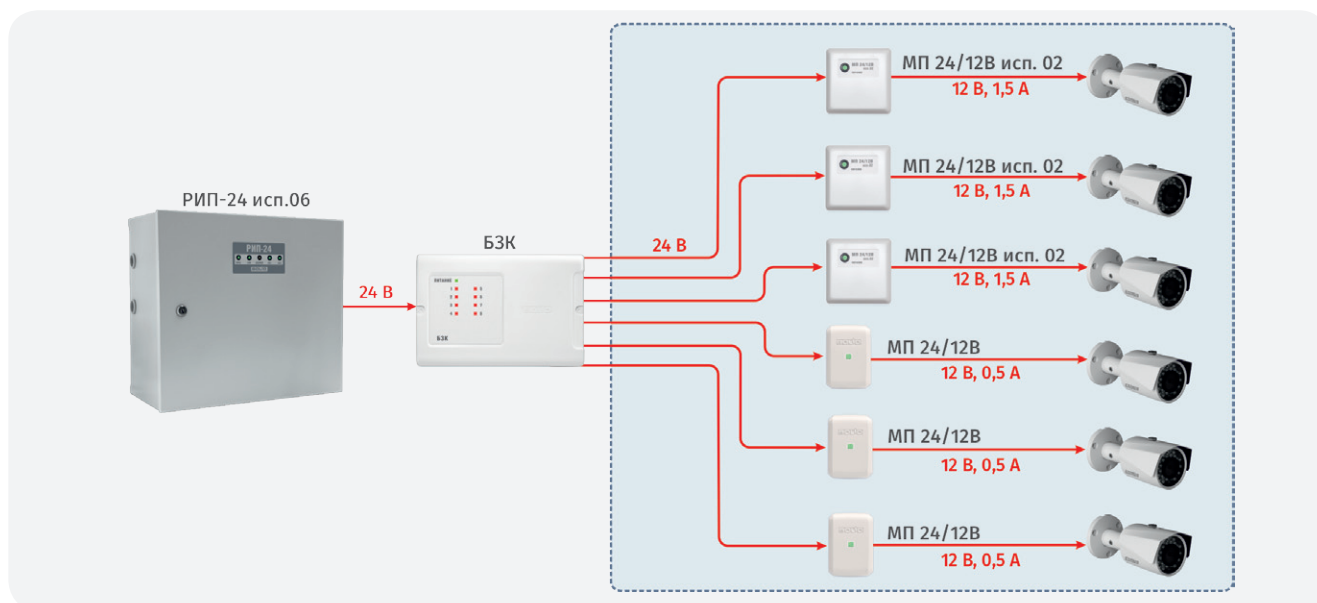
Рисунок 75. Организация электропитания системы видеонаблюдения
