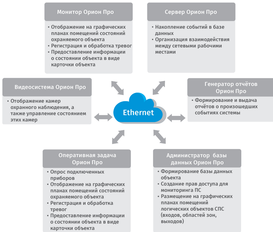
Рисунок 12. Функционал модулей программного обеспечения
