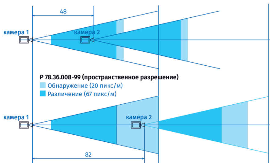
Рисунок 78. Варианты перекрытий зон обзора на протяженном периметре
