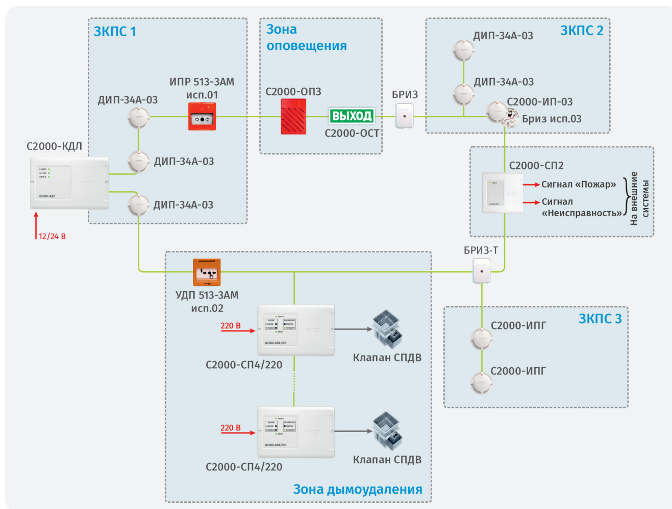
Рисунок 33. Структурная схема организации ДПЛС в СПА
