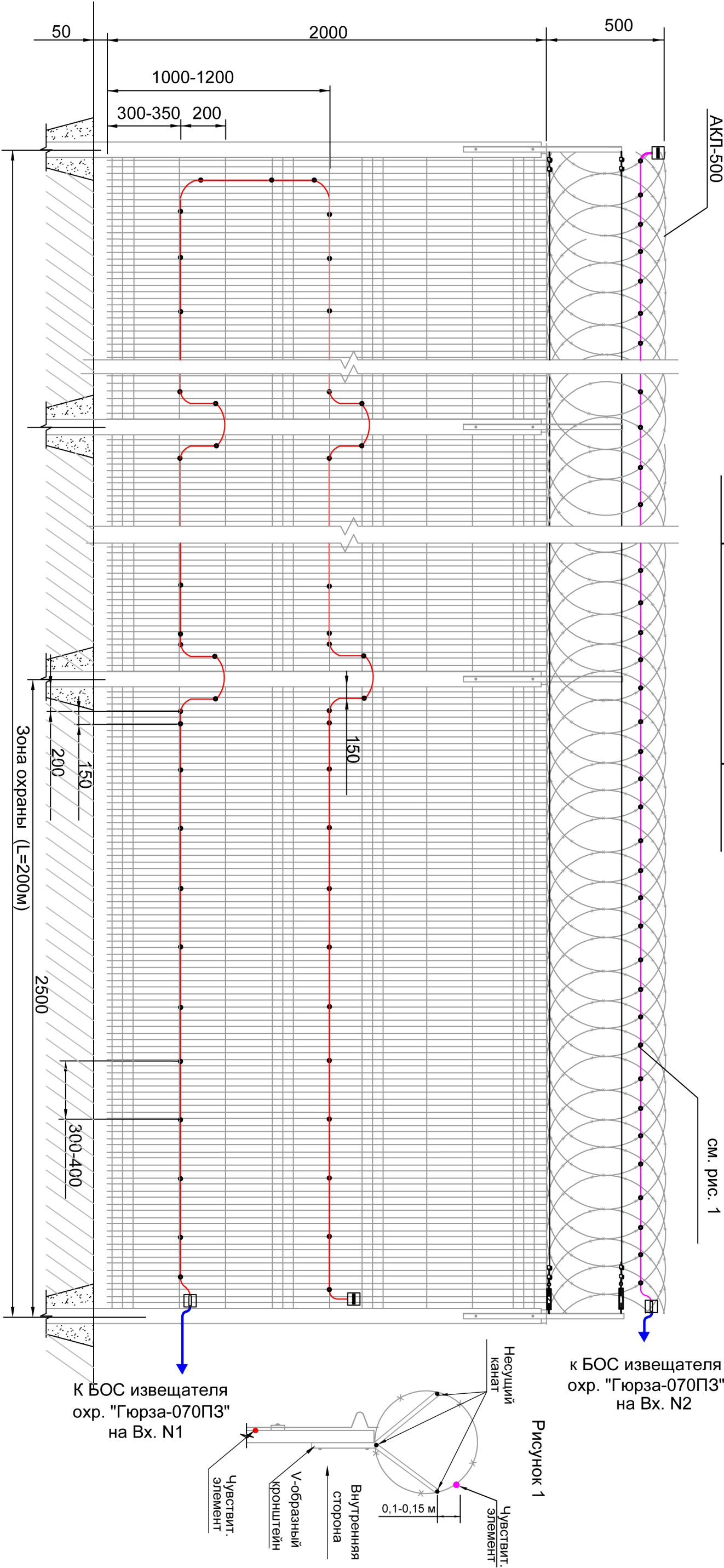
Спецификация на одну зону охраны длиной 200 м
