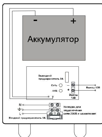
Схема подключения источника согласно рис. 1
