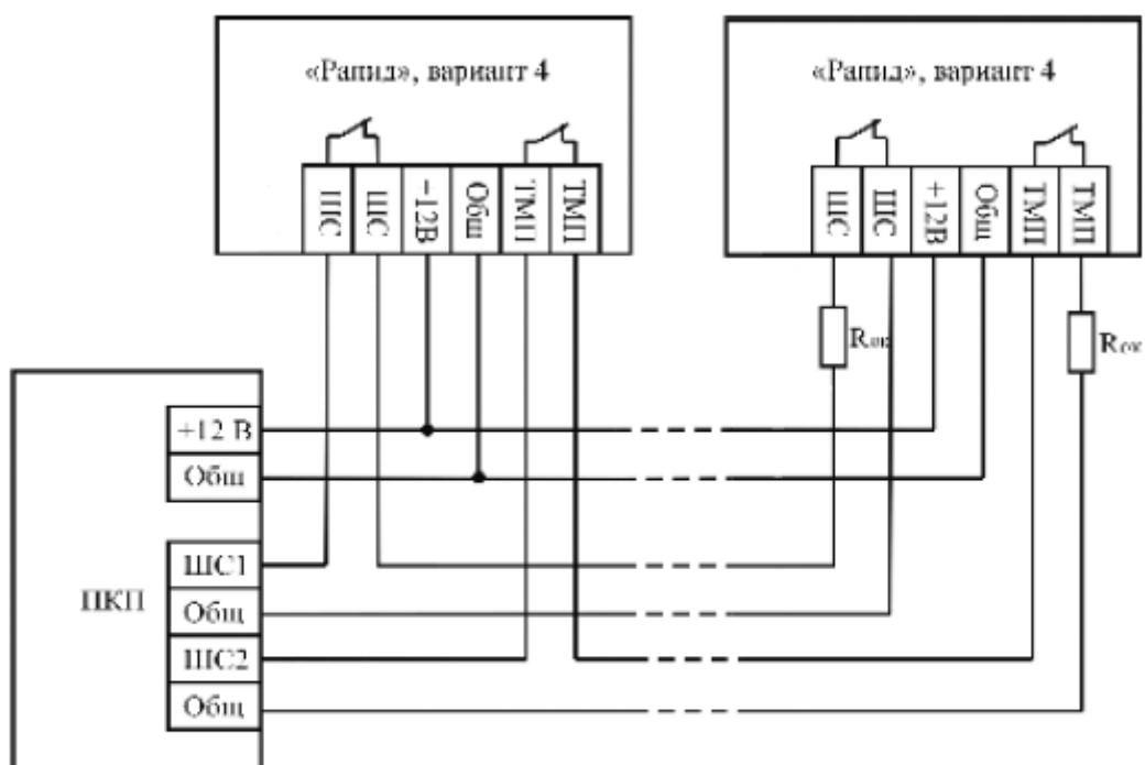
Рис. 2 Схема подключения извещателей
