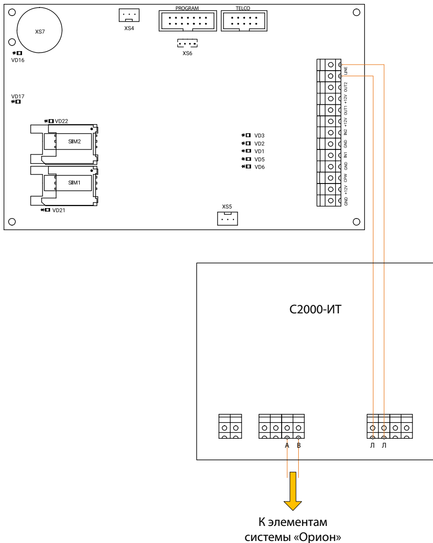
Рисунок 13. Схема подключения информатора телефонного C2000-ИТ
