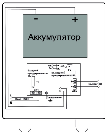
Схема подключения рис. 1
