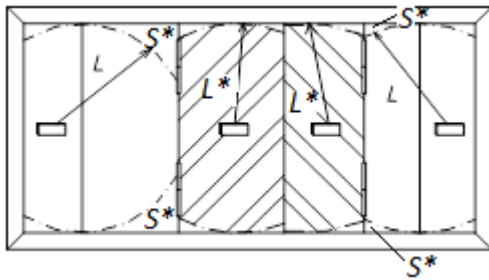
Рисунок 5. Защита немонолитной конструкции. ( S^* < 0,1 \text{ м}^2 , L < L^* )
