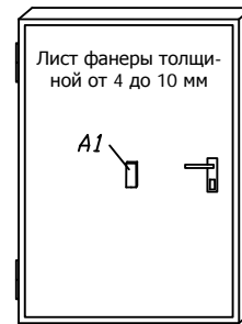
Рисунок 6. Защита деревянной пустотелой двери
