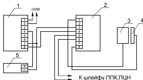
Схема подключения извещателя с экраном.
