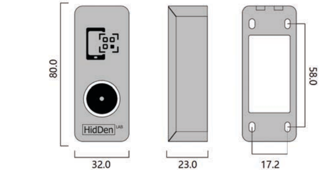
Рис.1 Габариты изделия.
