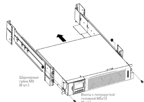
Рис. 4 Крепление передней части шкафа
