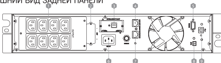
Вид сзади 1-1.5 кВА(С/Н)
