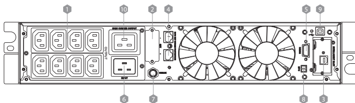
Вид сзади 3 кВА(С/Н)
