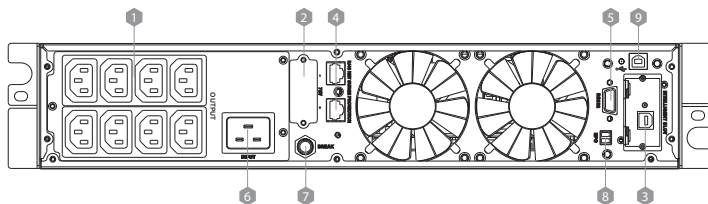
Вид сзади 2 кВА(С/Н)
