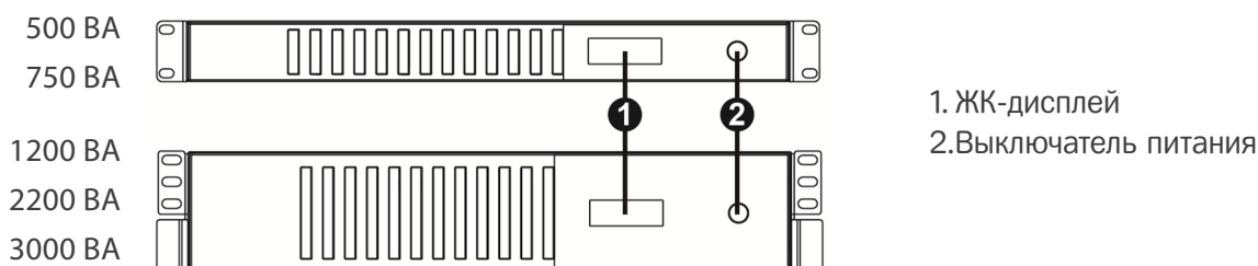
Рис. 2-1 Вид спереди
