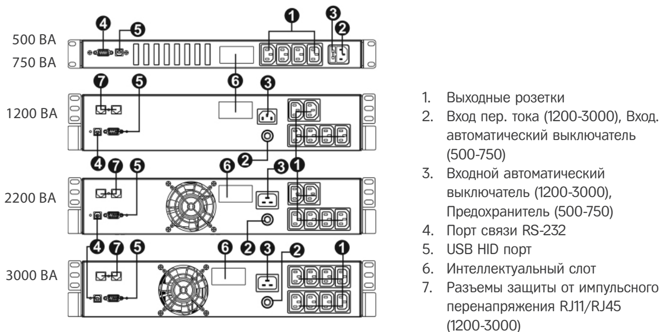
Рис. 2-3 Вид сзади
