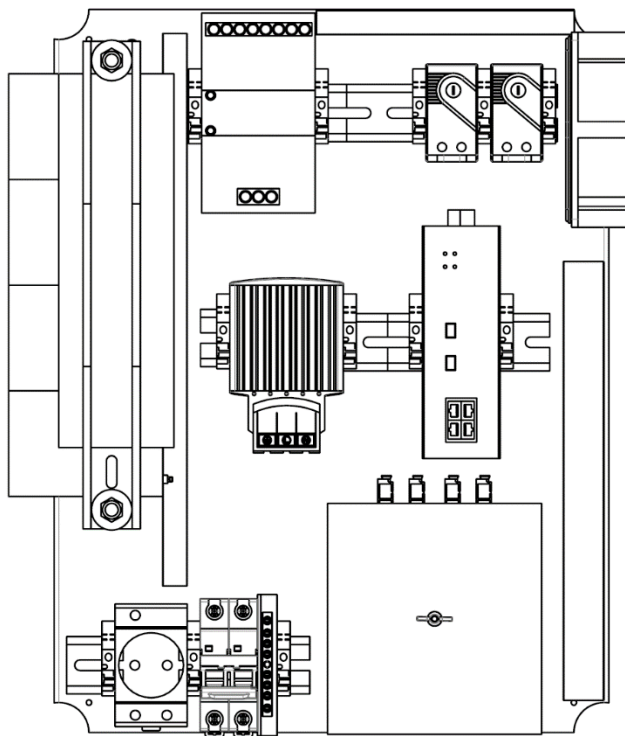
Рисунок 1 – Устройство шкафа
