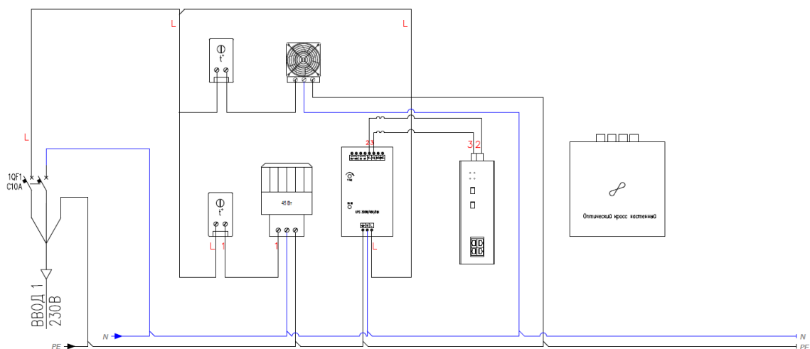
Рисунок 1 – Устройство шкафа
