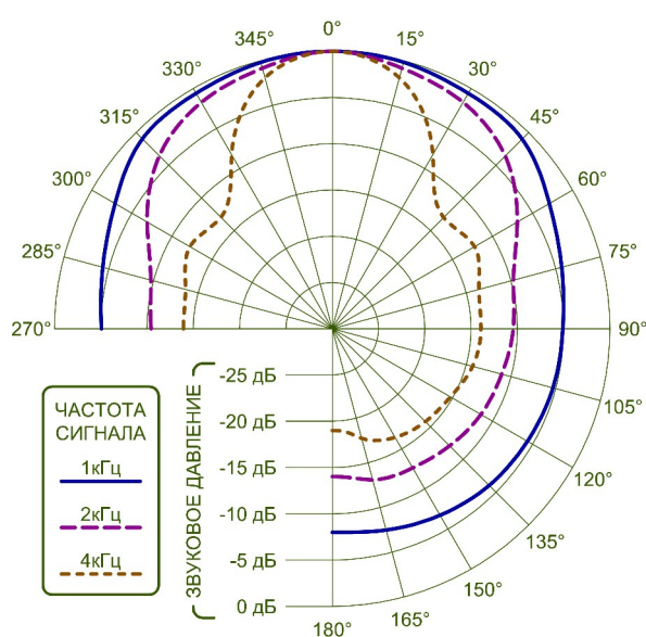
Диаграмма направленности АСР-20.2.4 исп.3 при вертикальной установке
