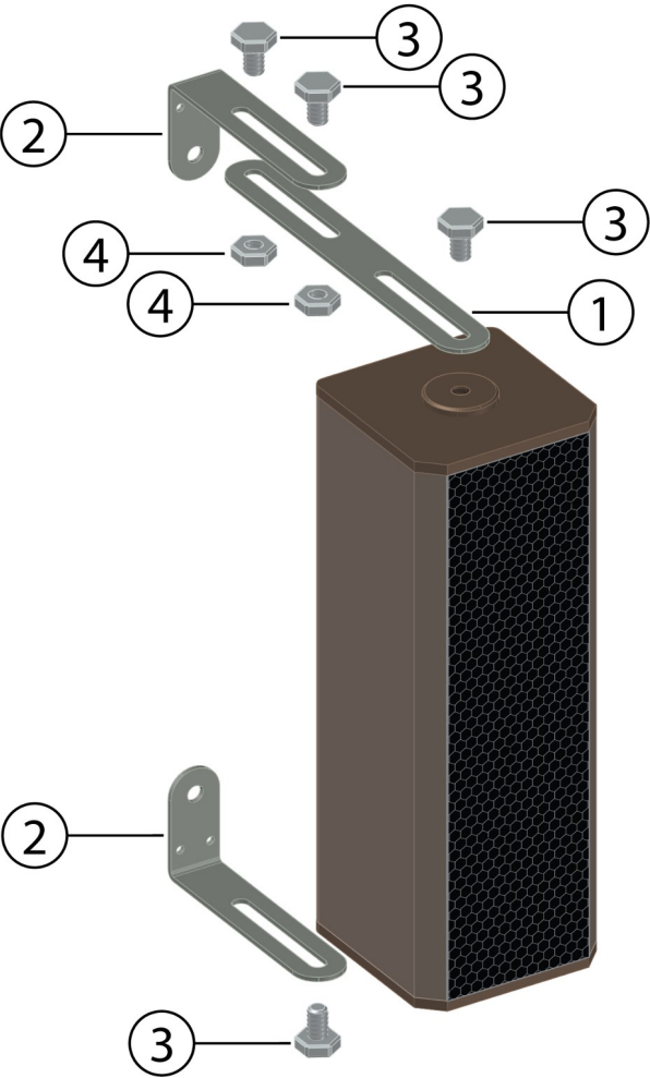
Рис.3 Комплект крепежных принадлежностей и установка крепежа БА
