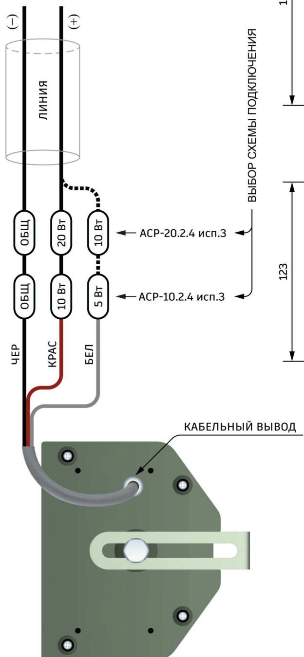
Рис.2 Габаритные, установочные размеры и схема подключения БА
