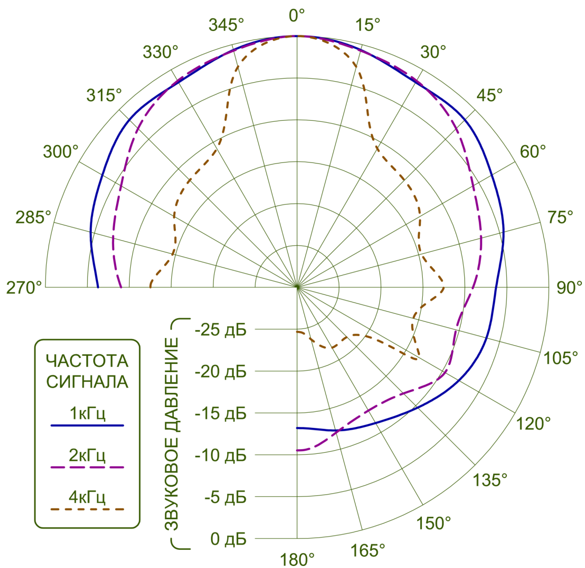
Рис.1 Характеристика направленности блоков акустических.
