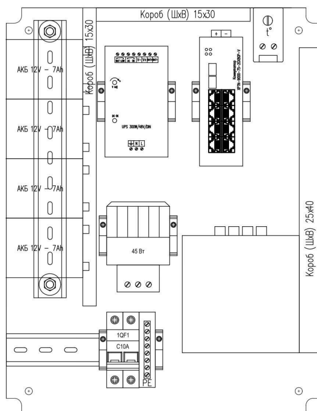
Рисунок 1 – Устройство шкафа
