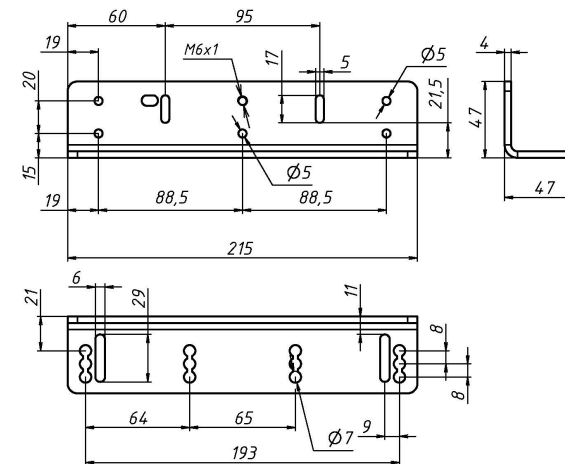
Рисунок 6 - L-уголок AL-350FB-M
