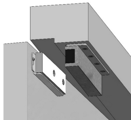
Рисунок 3 – Варианты установки корпуса замка на пластине
