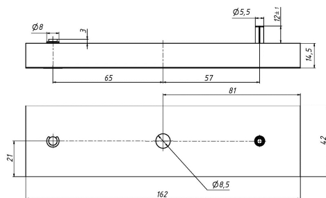
Рисунок 9 - Якорь
